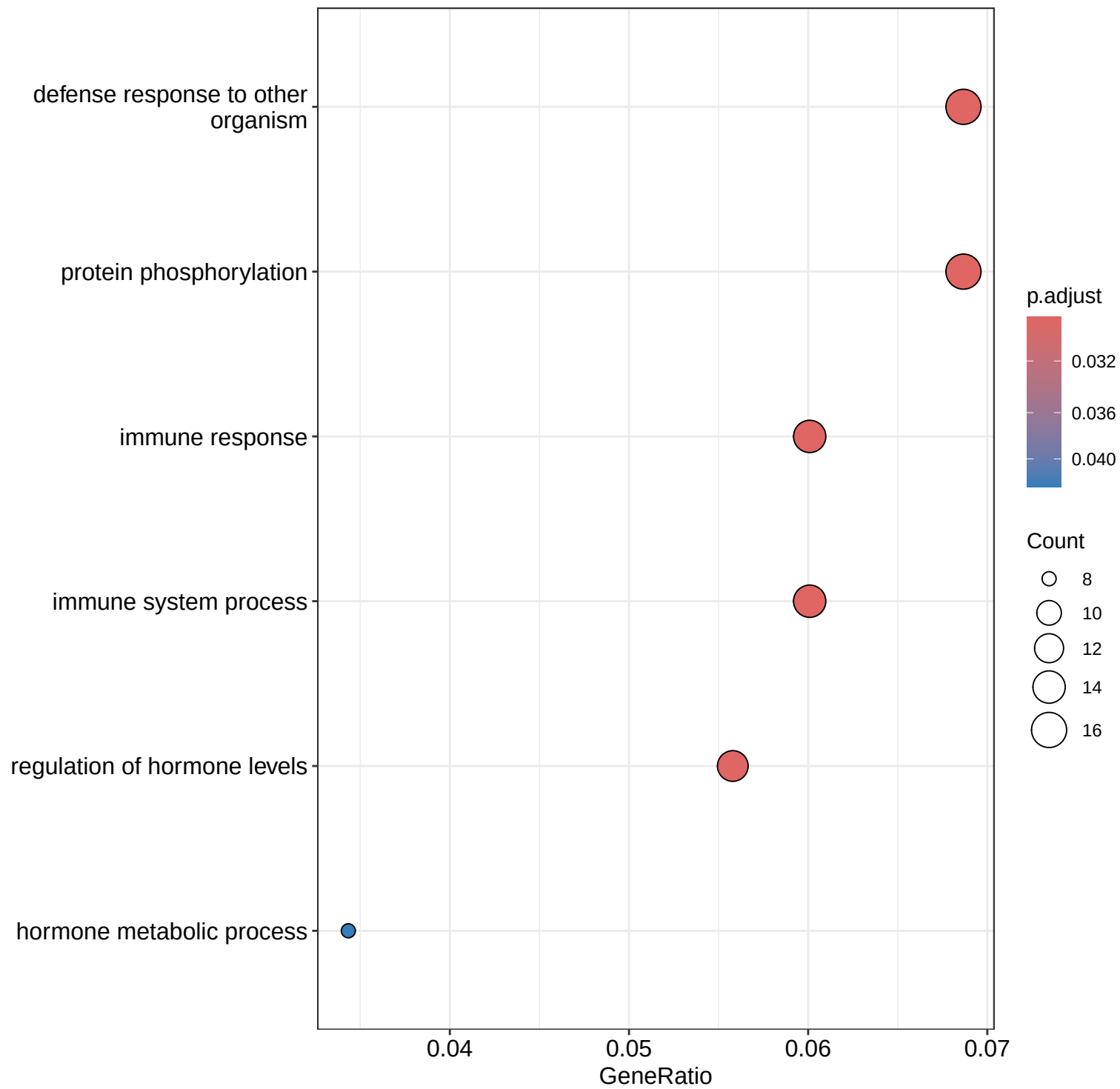
GO:BP up — D130_Root_FlightVsGround
