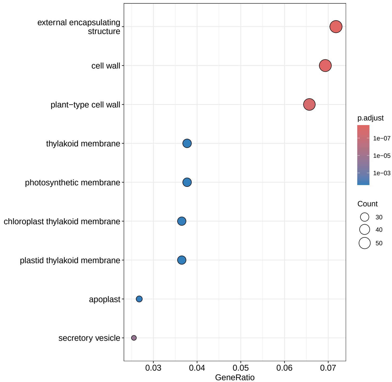
GO:CC all — D130_Shoot_FlightVsGround
