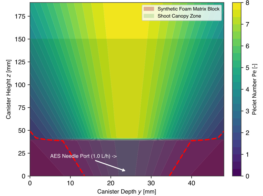
b PGC Canister Péclet Number ( Pe = uL/D )
