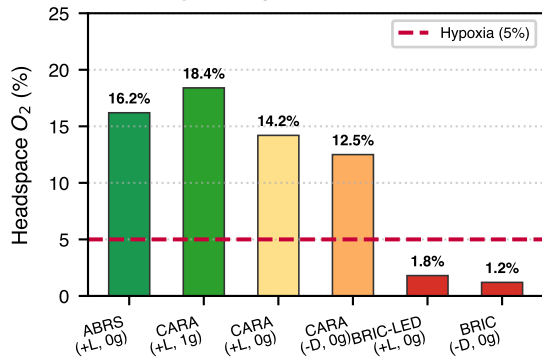
c Headspace Equilibrium O_2 (%)
