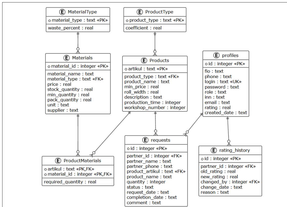
Рисунок 2.4 – ERD-диаграмма таблиц
