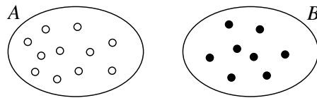
Slika 4.2: Princip zbira: |A \cup B| = |A| + |B| = 11 + 8 = 19
