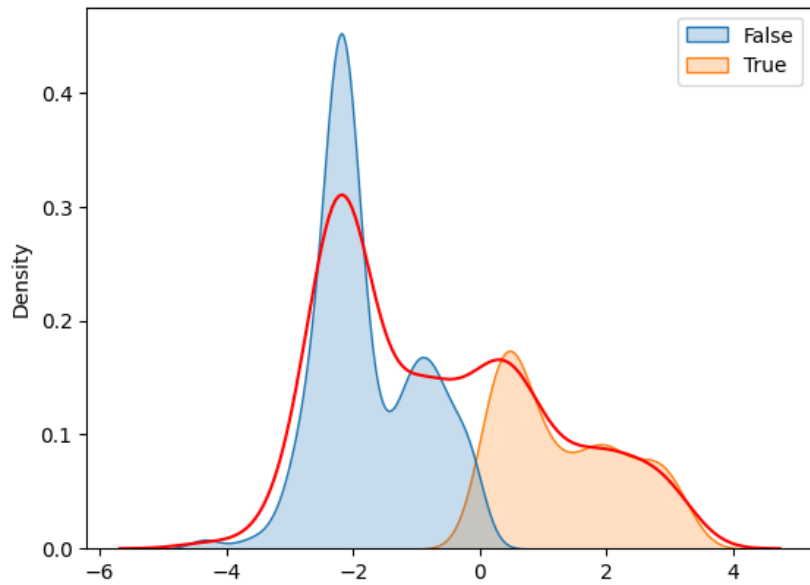
Figura 25: Densidades de la predicción usando el umbral de 0,5
