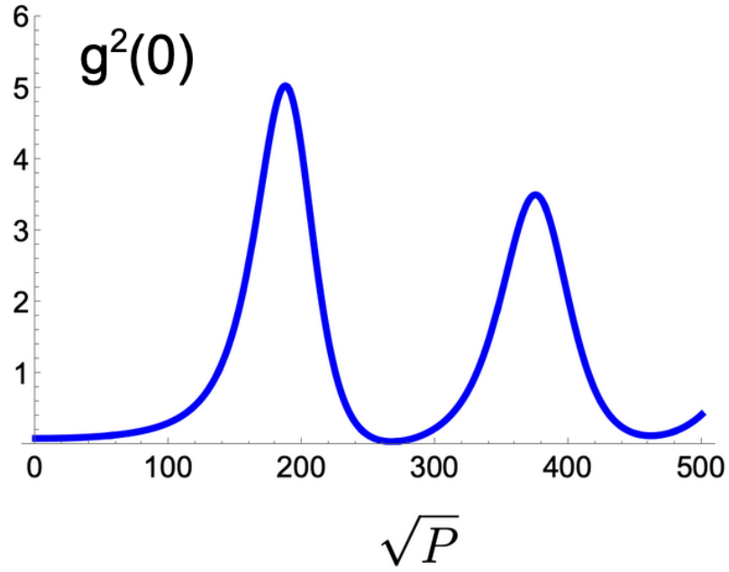
Рис. 9: Нормированная корреляционная функция второго порядка g^{(2)}(0) в зависимости от \sqrt{P} . Пики вблизи \sqrt{P} \approx 200 и 380 (значения g^{(2)}(0) \approx 5 и 3.5 ) указывают на суперпуассоновскую статистику фотонов, характерную для режима многофотонного испускания. В точках нечётных \pi -накачек g^{(2)}(0) \rightarrow 0 . Параметры: \tau_p = 16 пс, B = 3 Тл, T = 1 К.
