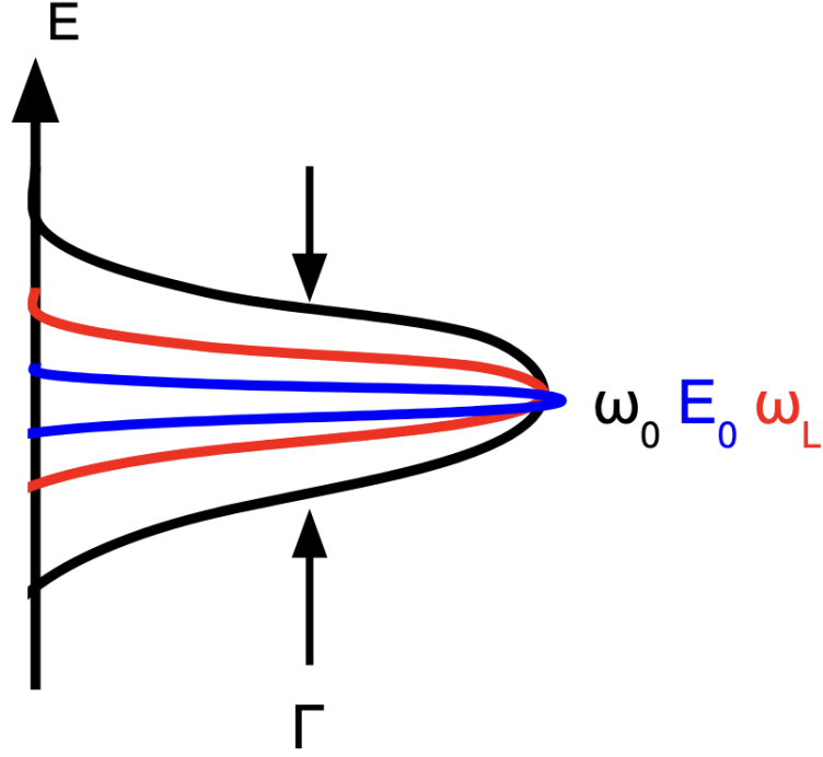
Рис. 1: Схема задачи с резонансным возбуждением [1]: лазер, частота резонатора \omega_0 и трионный переход E_0 совпадают. Накачка в H -поляризации, детектирование только в V -поляризации (кросс-поляризационная фильтрация). \Gamma — ширина микторезонатора.
