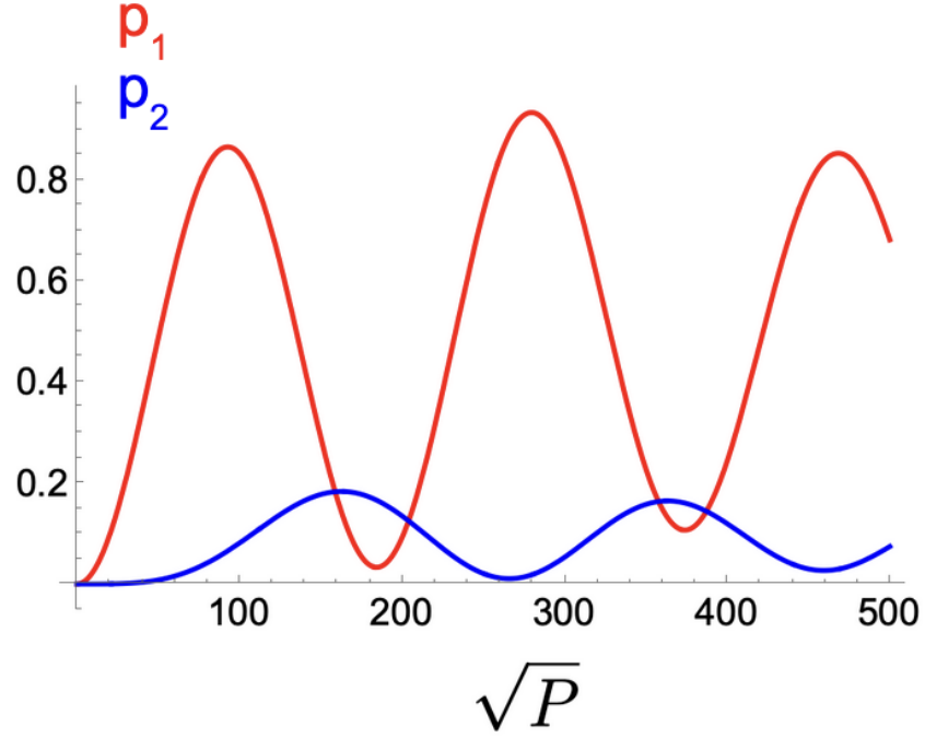
Рис. 7: Вероятности однофотонного ( p_1 , красная кривая) и двухфотонного ( p_2 , синяя кривая) выходных состояний в зависимости от \sqrt{P} — квадратного корня из мощности накачки. p_1 демонстрирует осцилляции Раби. Параметры: \tau_p = 16 пс, B = 3 Тл, T = 1 К.
