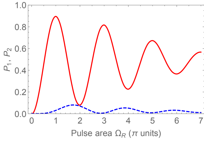
FIG. 2. p1p2
