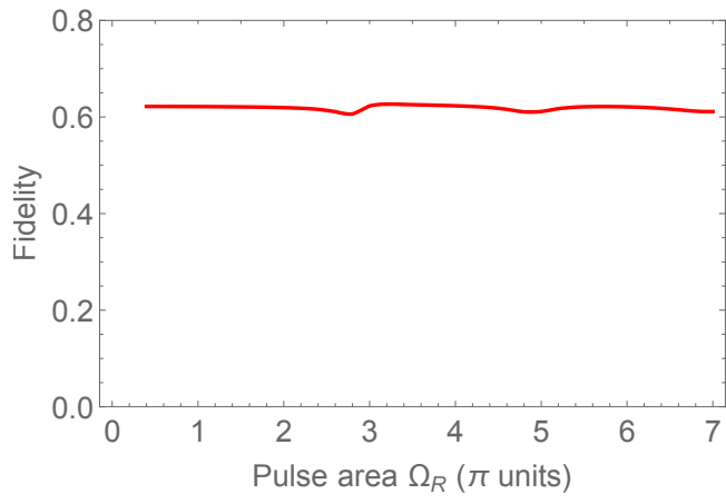
FIG. 5. fidelity
