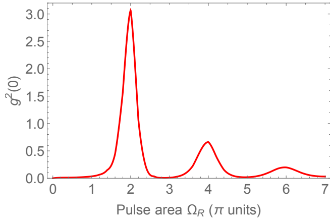
FIG. 3. g2(0)
