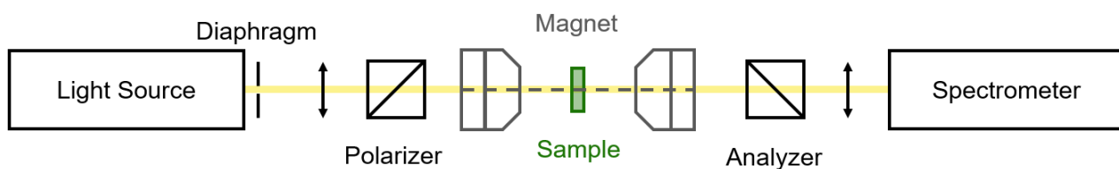
Рисунок 8 Схема установки магнитооптической спектроскопии
