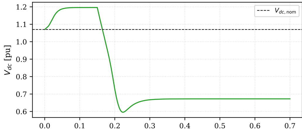
S4 — G: 1.0 → 0.3 pu
