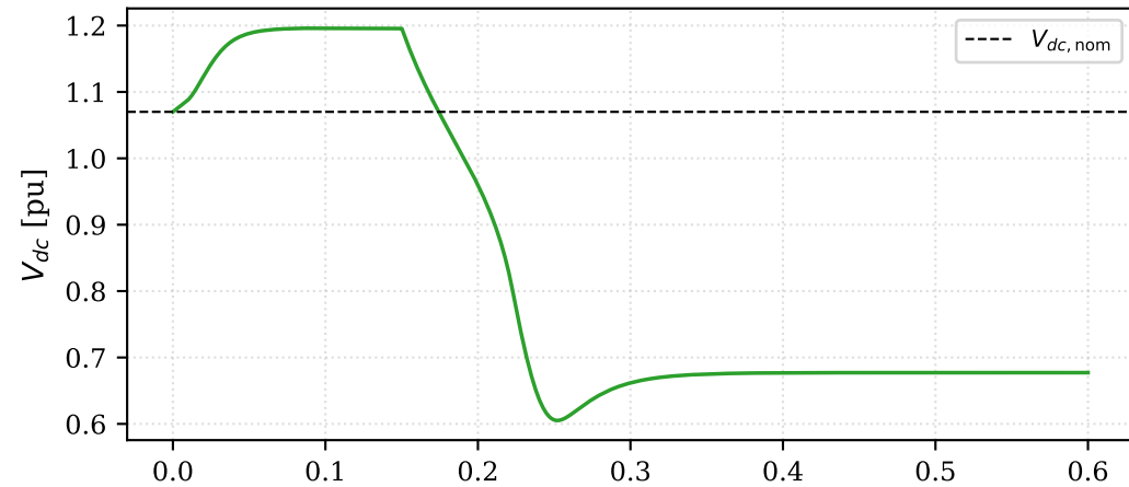
S3 — G: 1.0 → 0.5 pu
