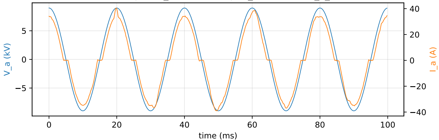
Scenario 06 (wang2020_default) — \alpha_{\text{true}}=0.30 , R_x=200\ \Omega
