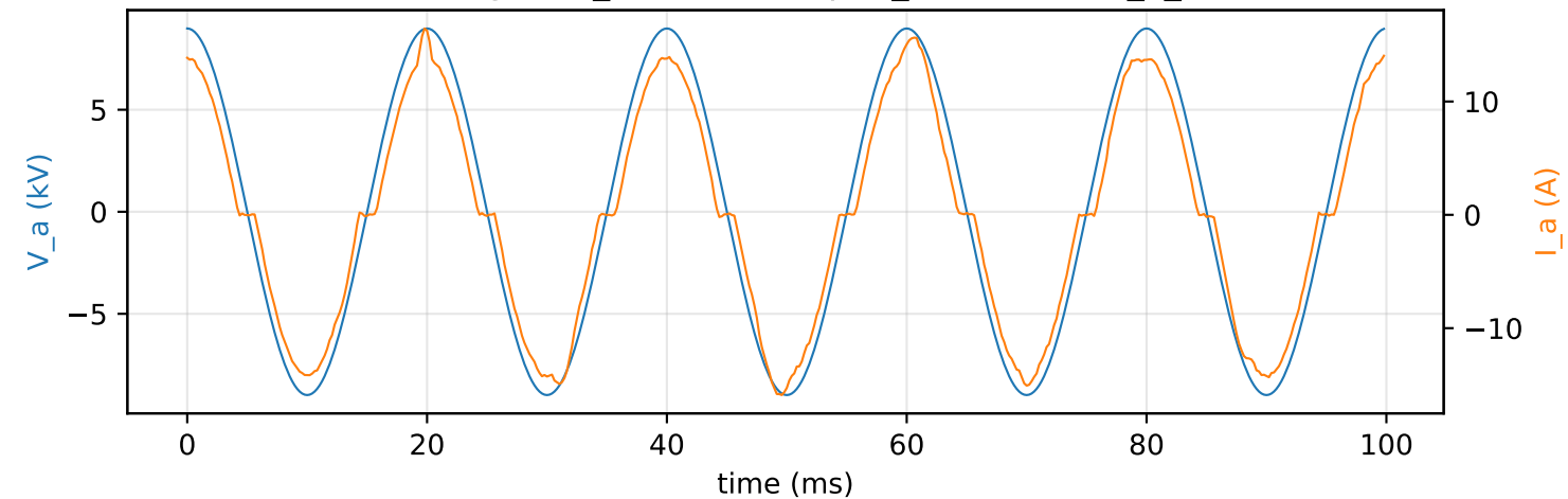
Scenario 07 (wang2020_default) — \alpha_{\text{true}}=0.30 , R_x=500\ \Omega
