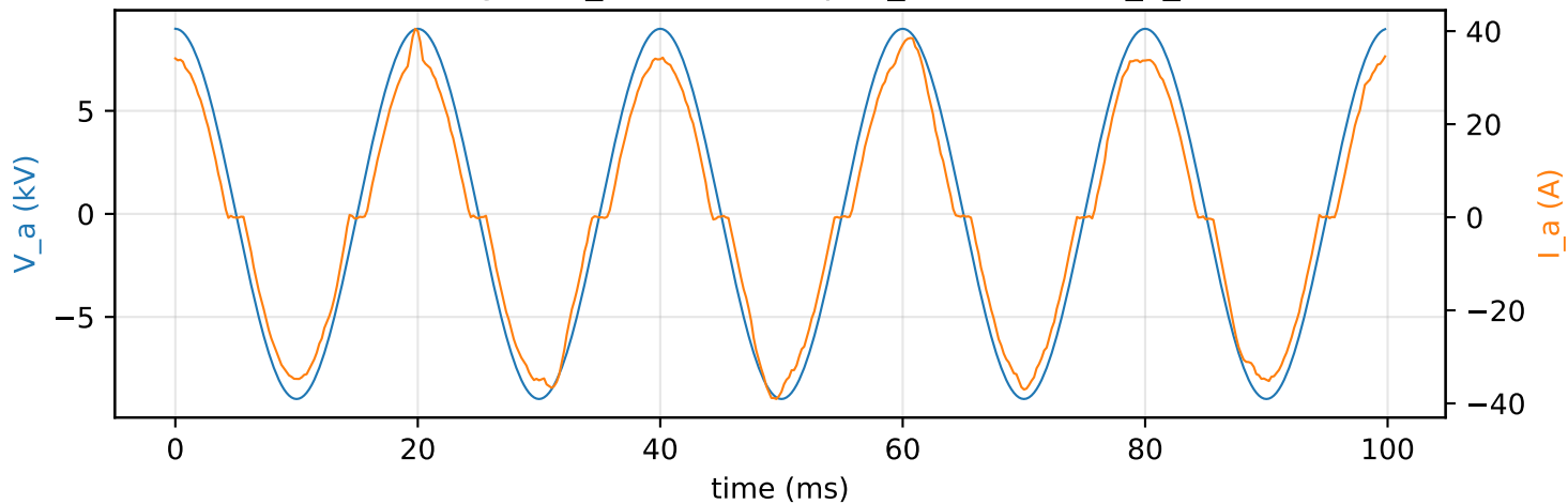
Scenario 11 (wang2020_default) — \alpha_{\text{true}}=0.50 , R_x_{\text{true}}=200\ \Omega
