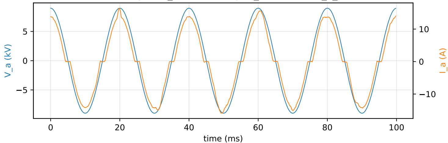
Scenario 12 (wang2020_default) — \alpha_{\text{true}}=0.50 , R_x_{\text{true}}=500\ \Omega
