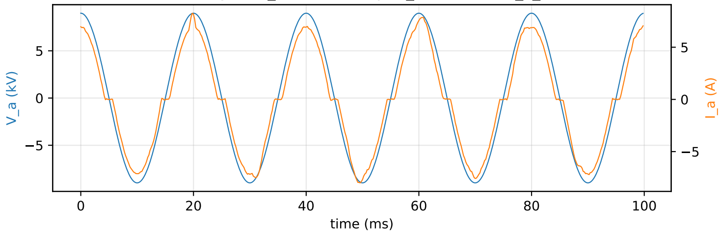
Scenario 13 (wang2020_default) — \alpha_{\text{true}}=0.50 , R_{\text{x\_true}}=1000\ \Omega
