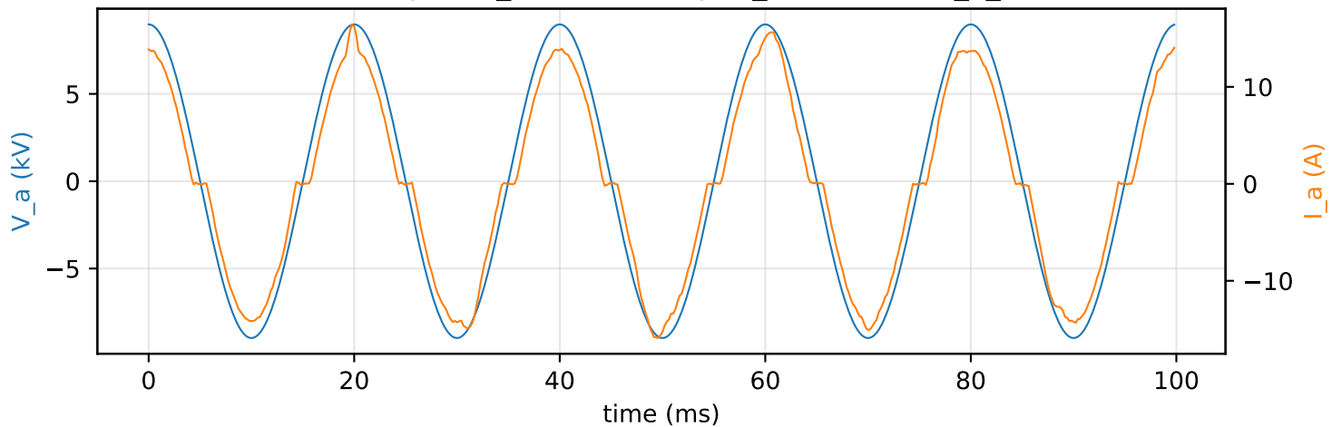
Scenario 17 (wang2020_default) — \alpha_{\text{true}}=0.70 , R_x_{\text{true}}=500\ \Omega
