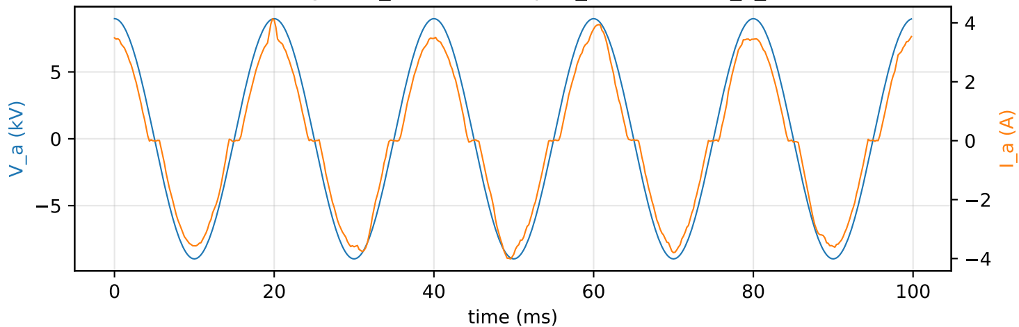
Scenario 19 (wang2020_default) — \alpha_{\text{true}}=0.70 , R_x_{\text{true}}=2000\ \Omega
