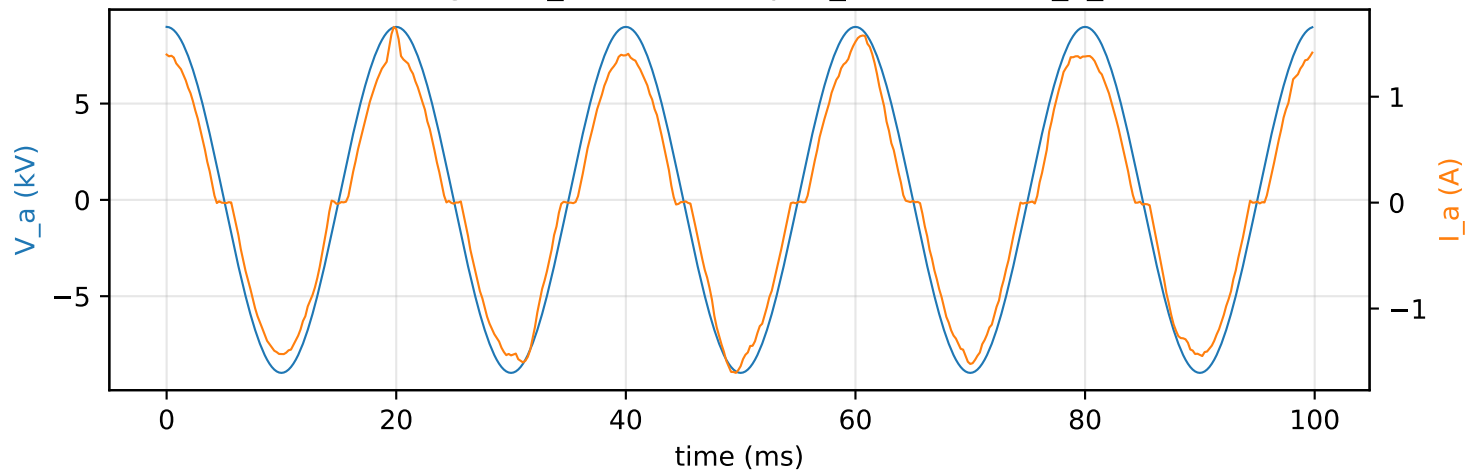
Scenario 20 (wang2020_default) — \alpha_{\text{true}}=0.70 , R_x_{\text{true}}=5000\ \Omega
