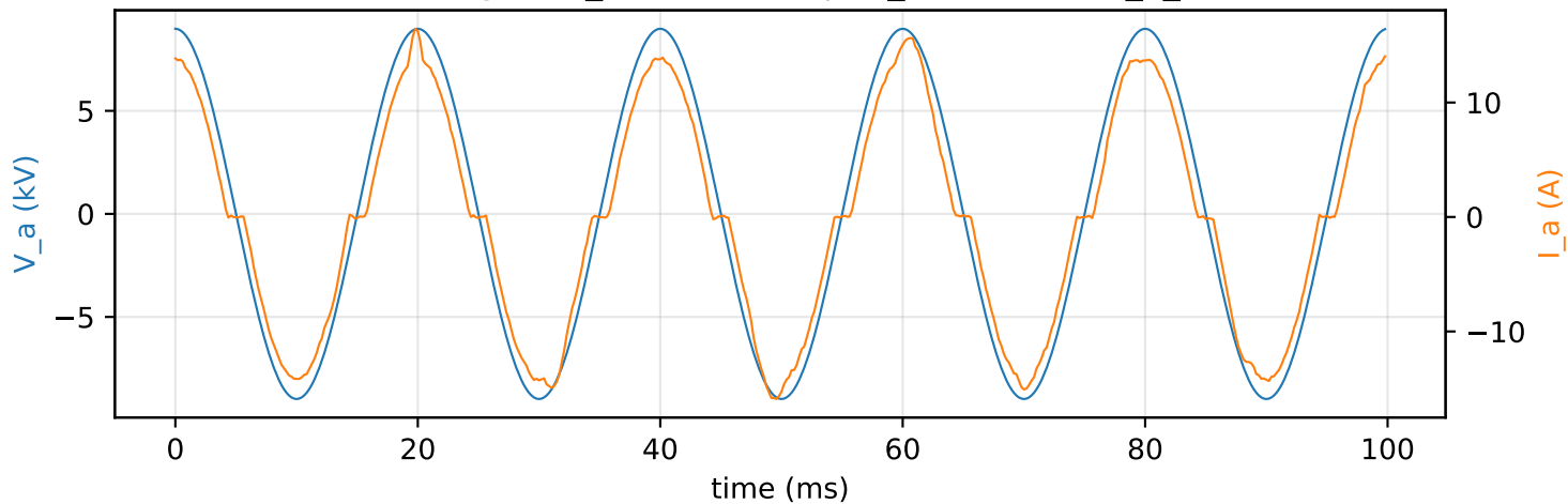
Scenario 22 (wang2020_default) — \alpha_{\text{true}}=0.90 , R_x_{\text{true}}=500\ \Omega
