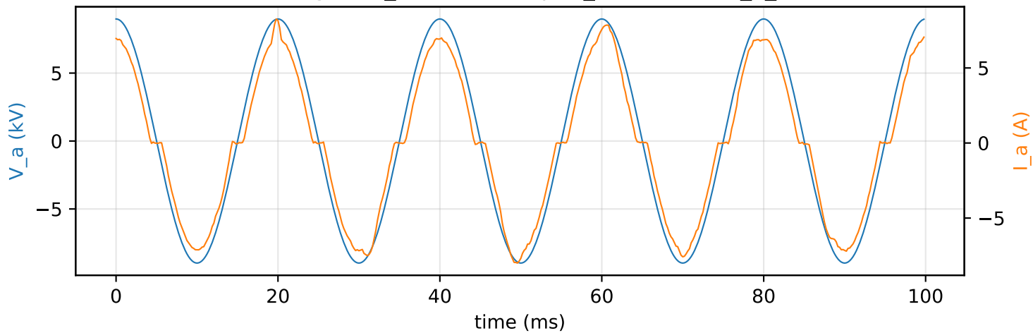
Scenario 23 (wang2020_default) — \alpha_{\text{true}}=0.90 , R_{\text{x\_true}}=1000\ \Omega
