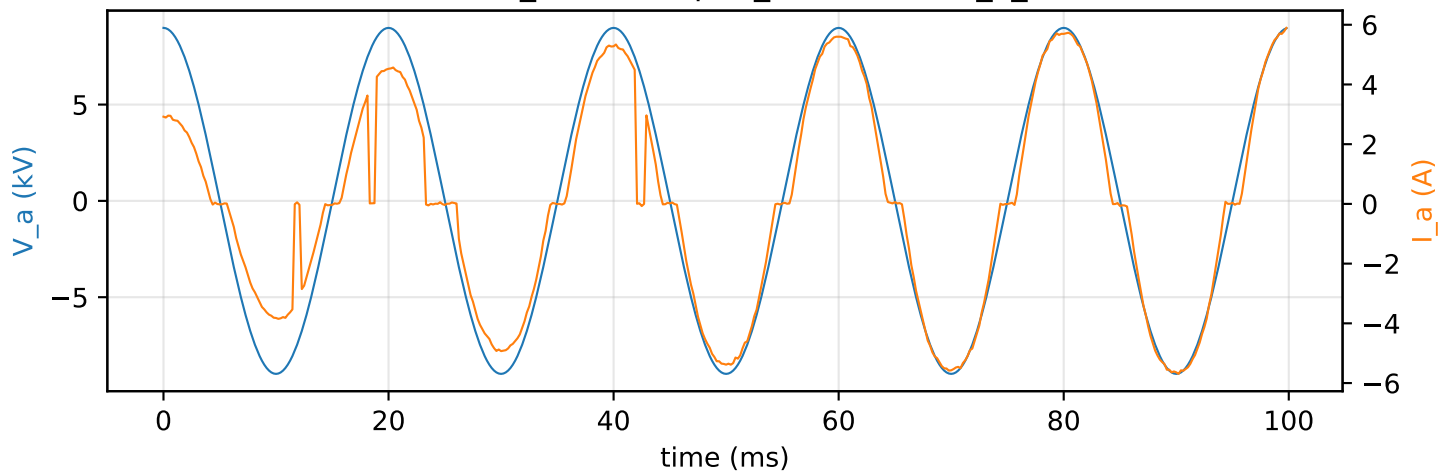
Scenario 28 (torres_tree) — \alpha_{\text{true}}=0.50 , R_{x\_true}=1000\ \Omega
