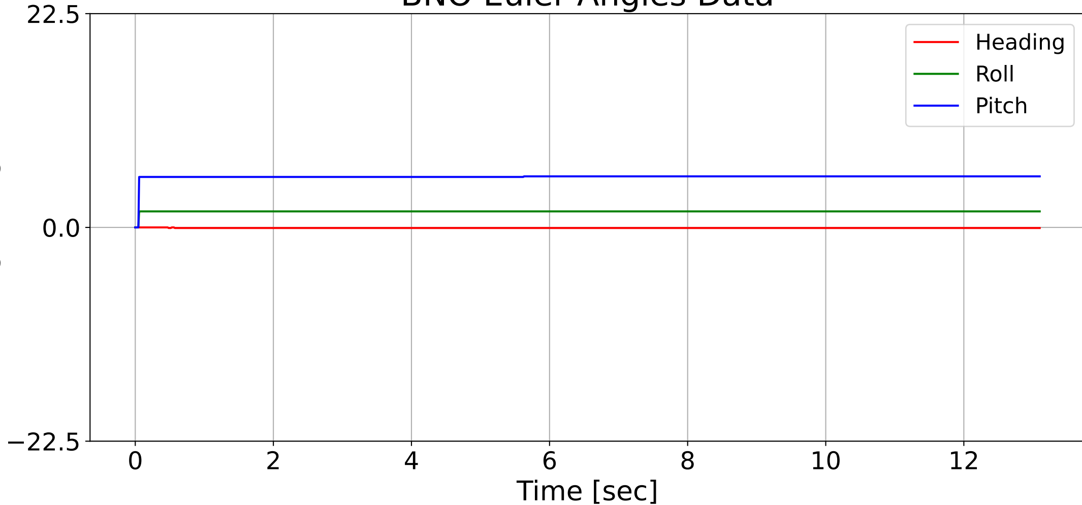
BNO Euler Angles Data
