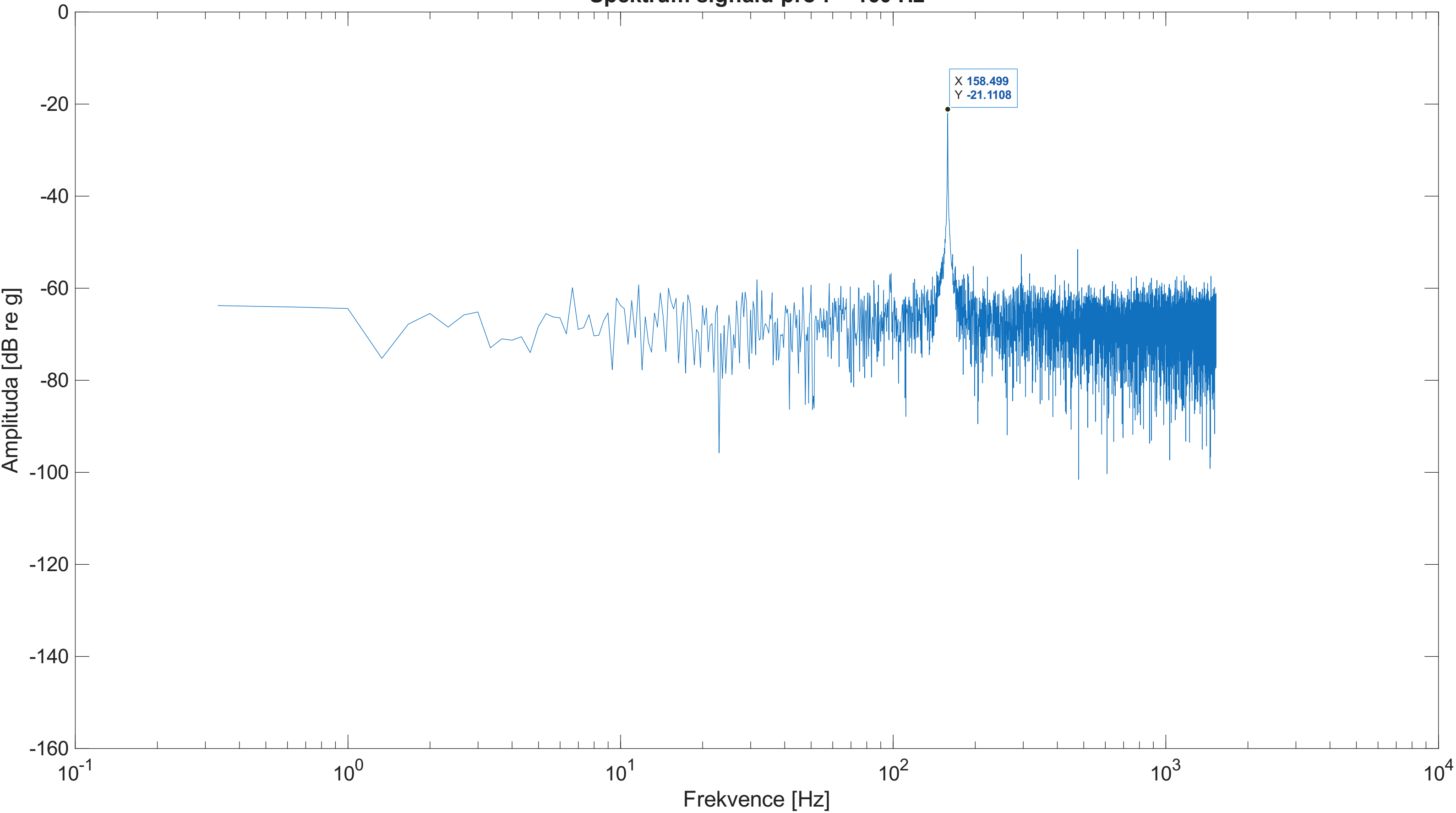
Spektrum signálu pro f = 160 Hz
