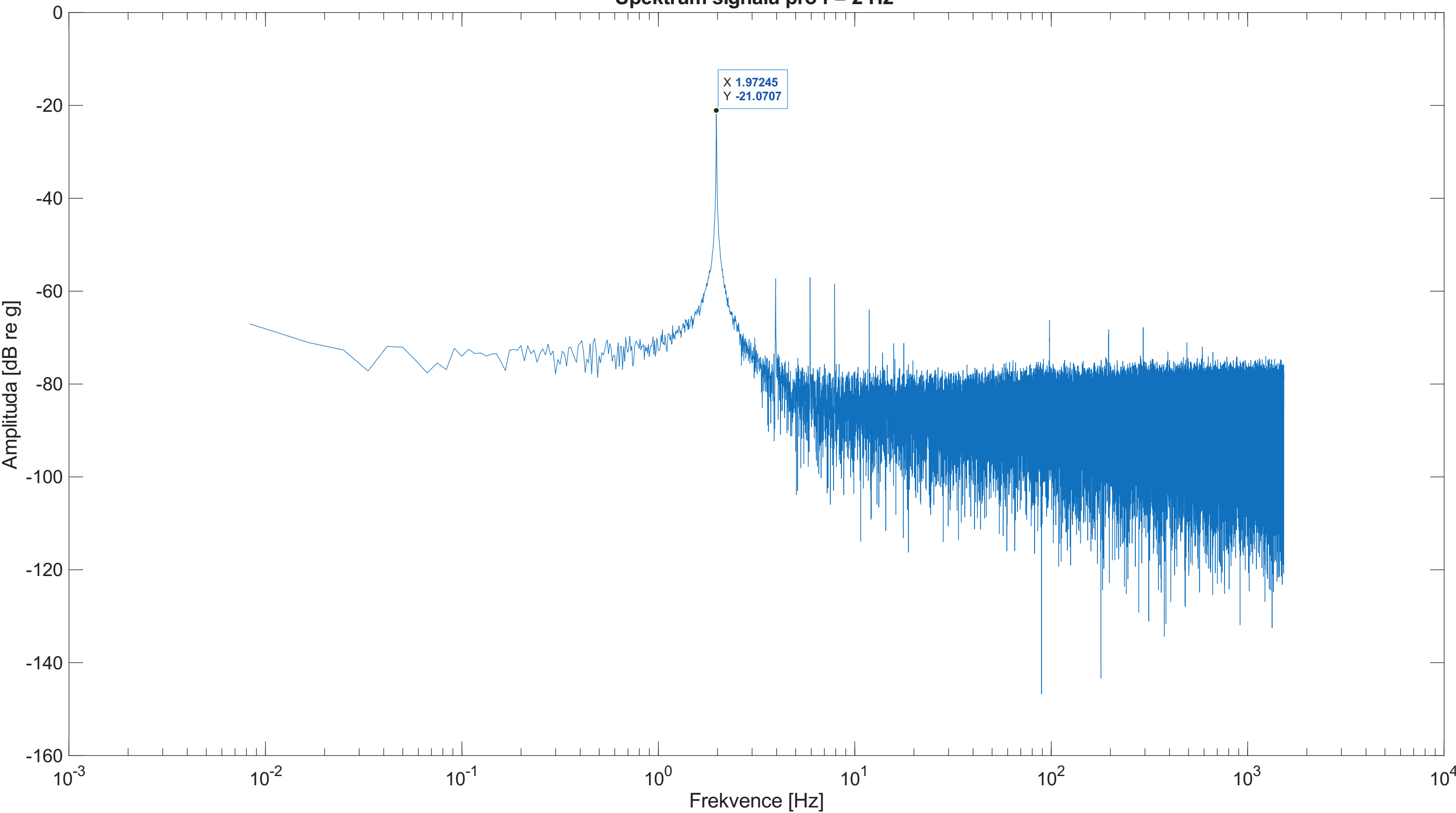
Spektrum signálu pro f = 2 Hz
