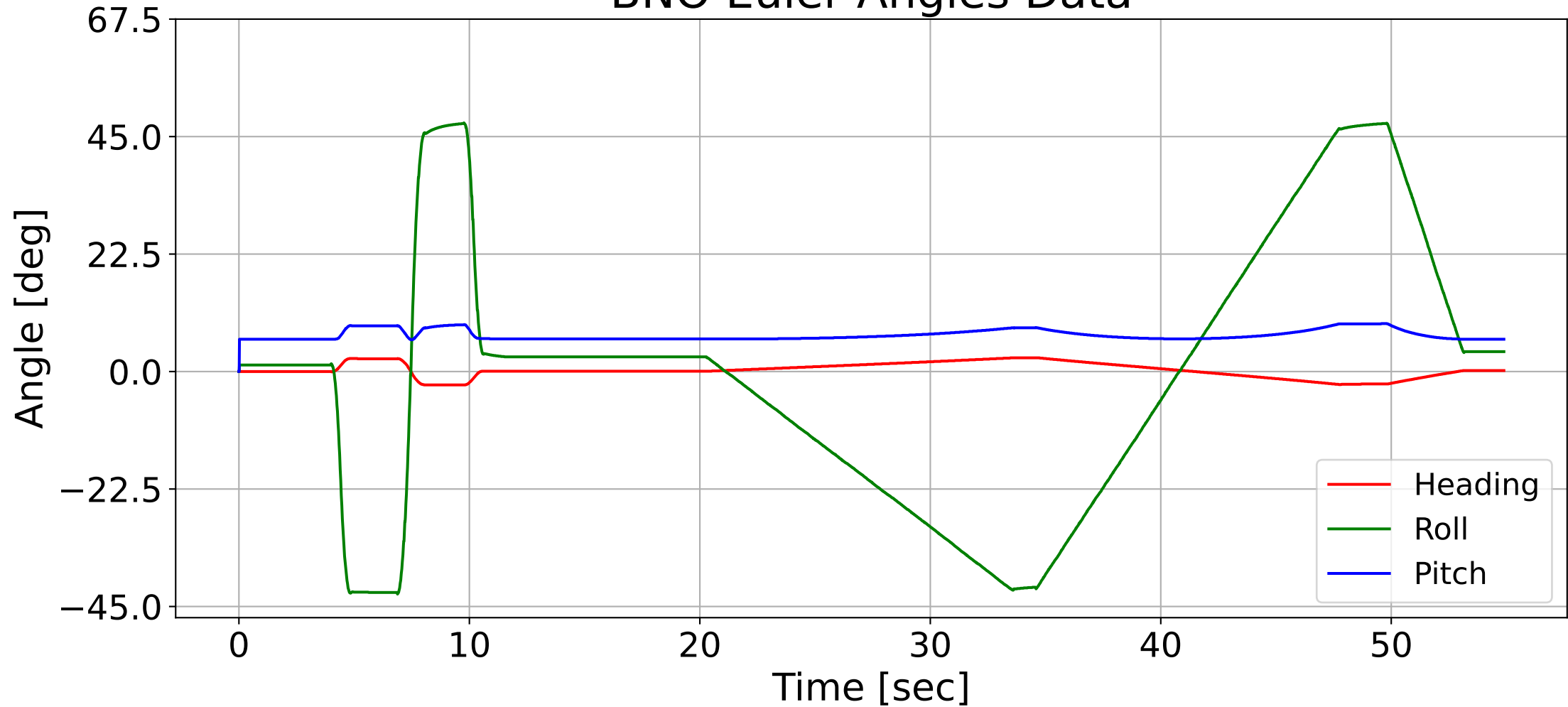
BNO Euler Angles Data
