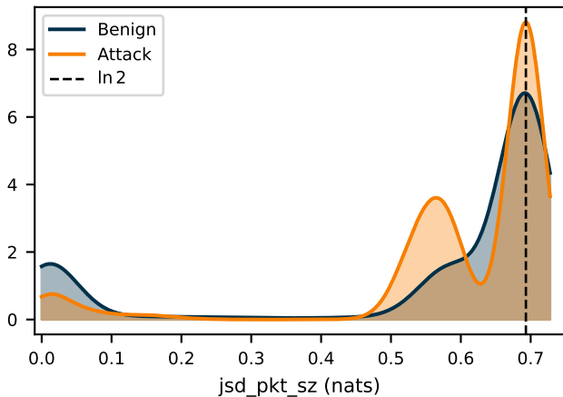
UNSW-NB15
