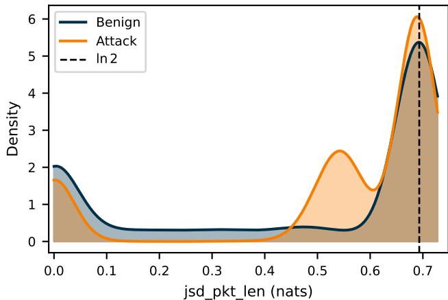
CICIDS-2017
