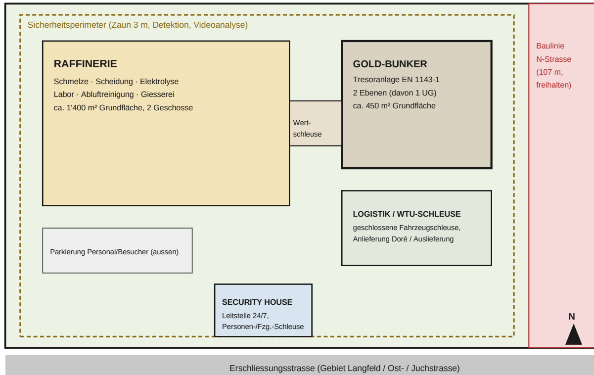
Parzelle 61522 · 6'434 m 2 (Schema, nicht massstäblich)
