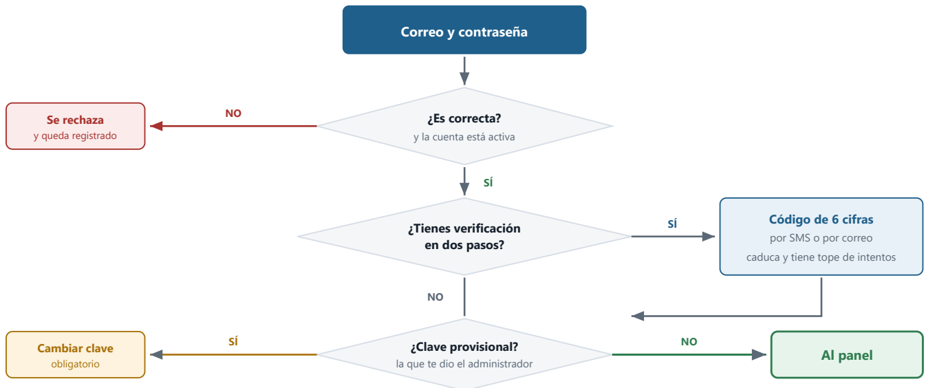
FIGURA 4 — Flujo de acceso, con sus dos desvíos.
