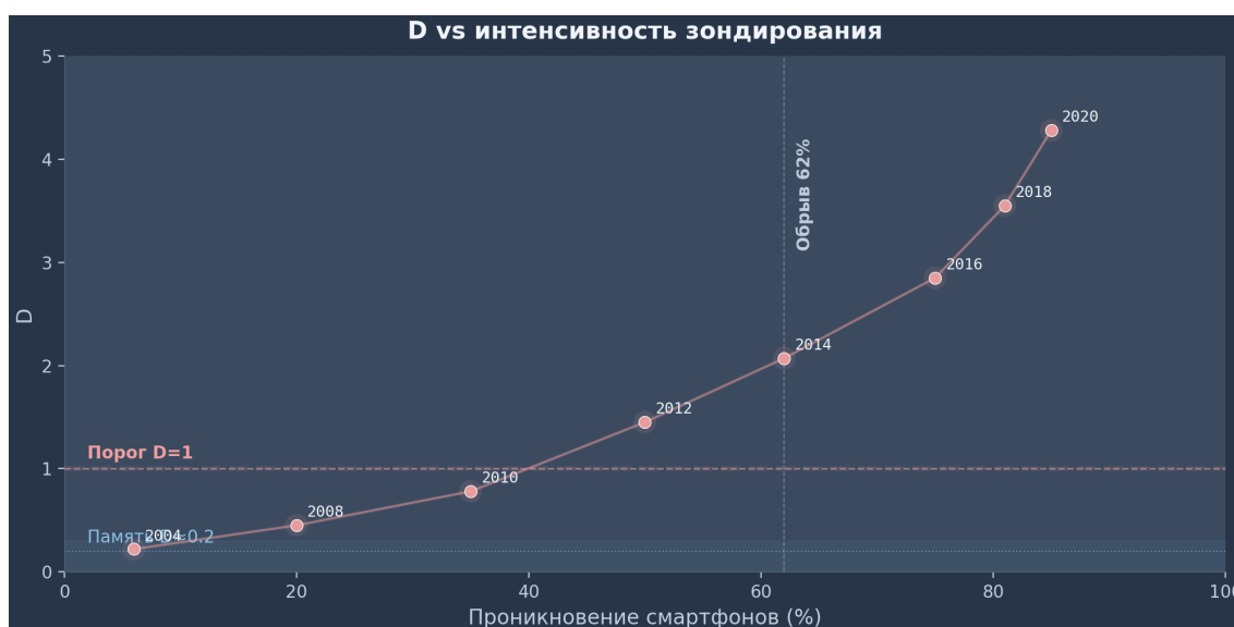
Рис. 2. D монотонно возрастает с проникновением смартфонов. Каждая точка — скользящее окно данных Глории Марк.
