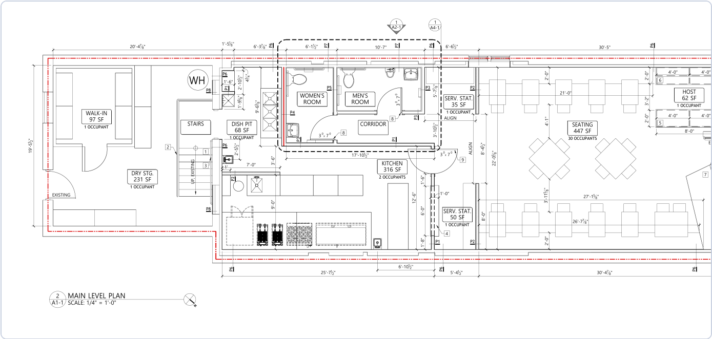
A1-1 Main Level Plan · Front/entrance = right (8th Avenue) · Back-of-house = left · Entrada = derecha · Área de servicio = izquierda
