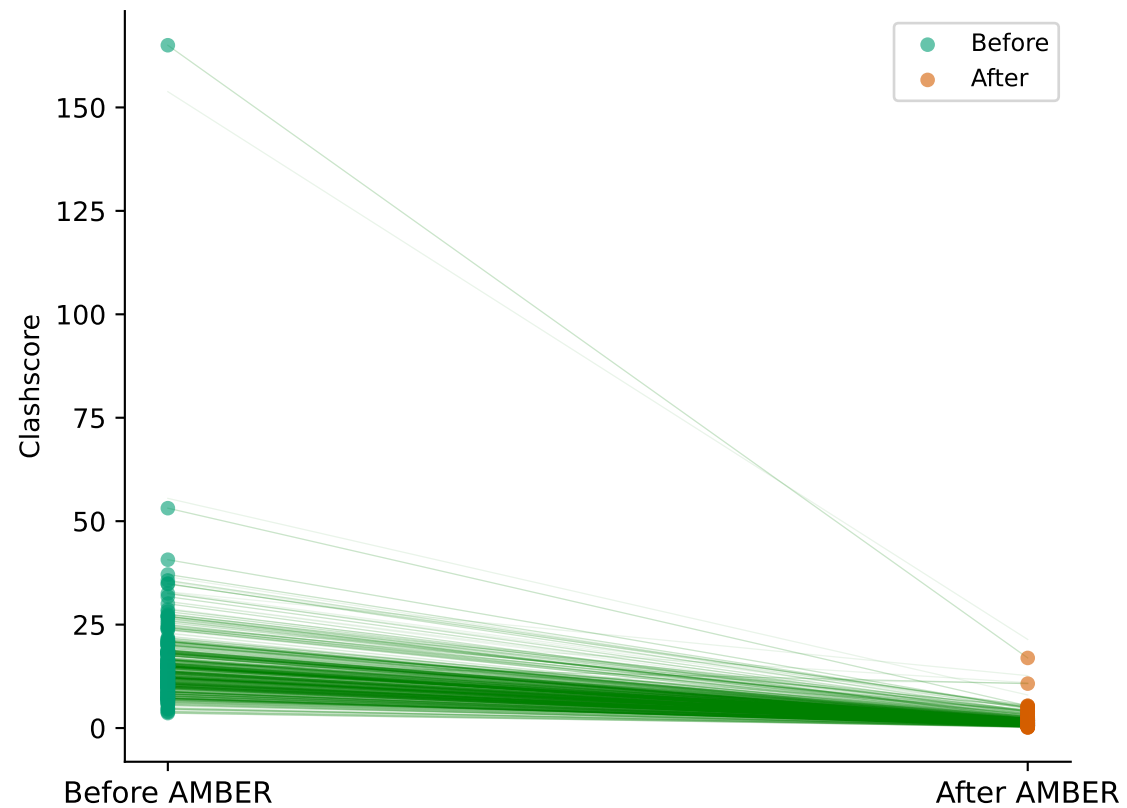
Boltz-1 → AMBER(Boltz)
