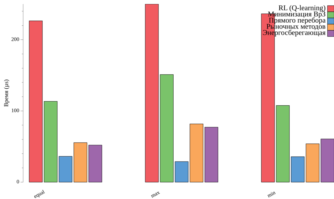
Рис. 4: Общее время выполнения
