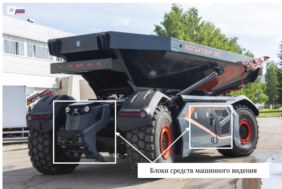
Рис. 2: Набор датчиков «Юпитер-30» ПАО «КАМАЗ»
