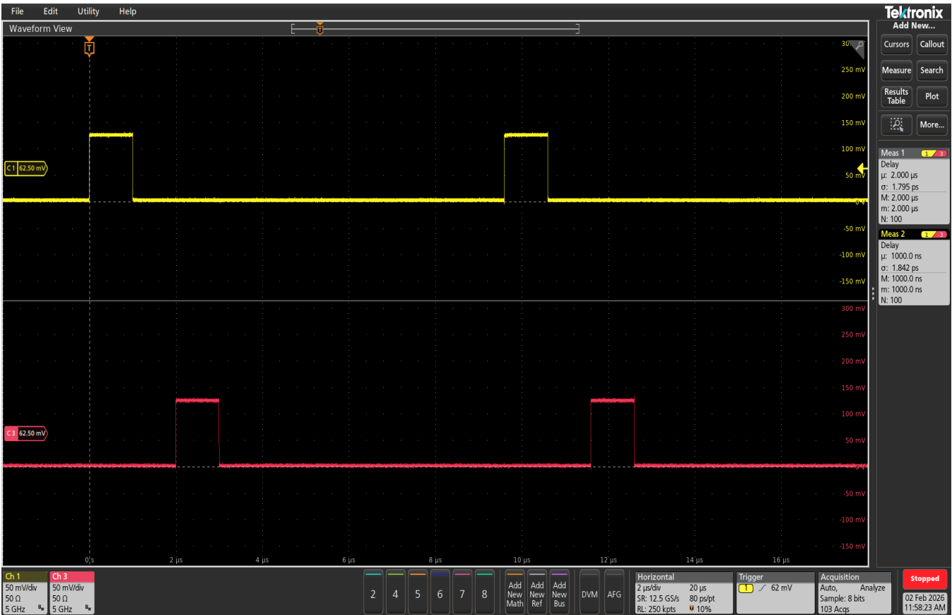
Test 1: delay_view.png
