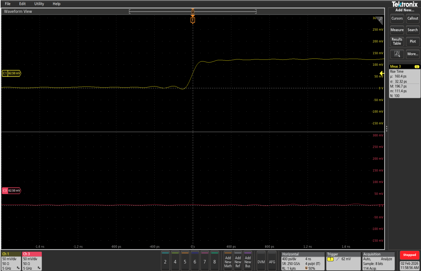
Test 3: rise_time_ch1.png
