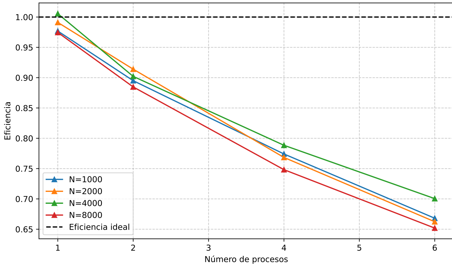
Matriz-vector: eficiencia
