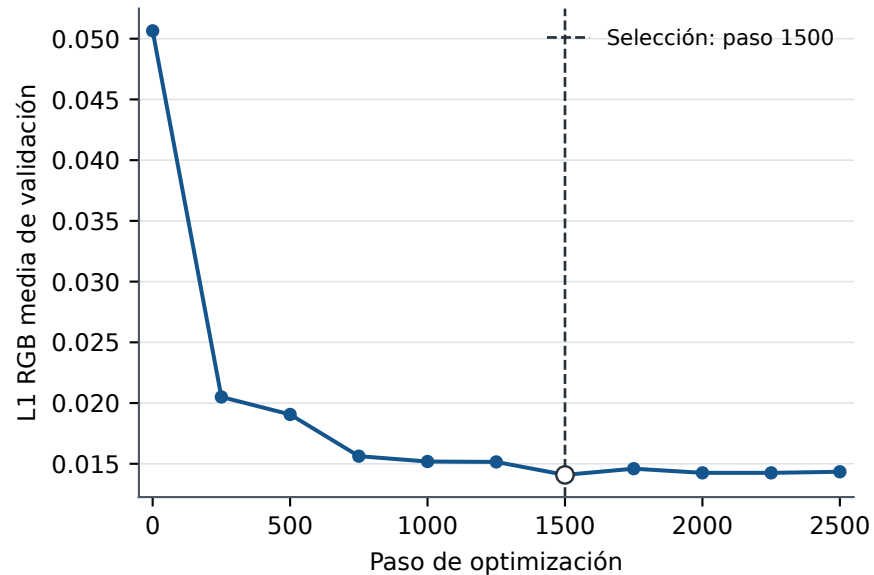
EDSR x2
