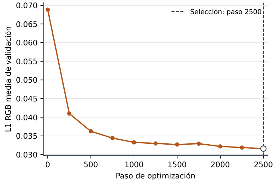
EDSR x4
