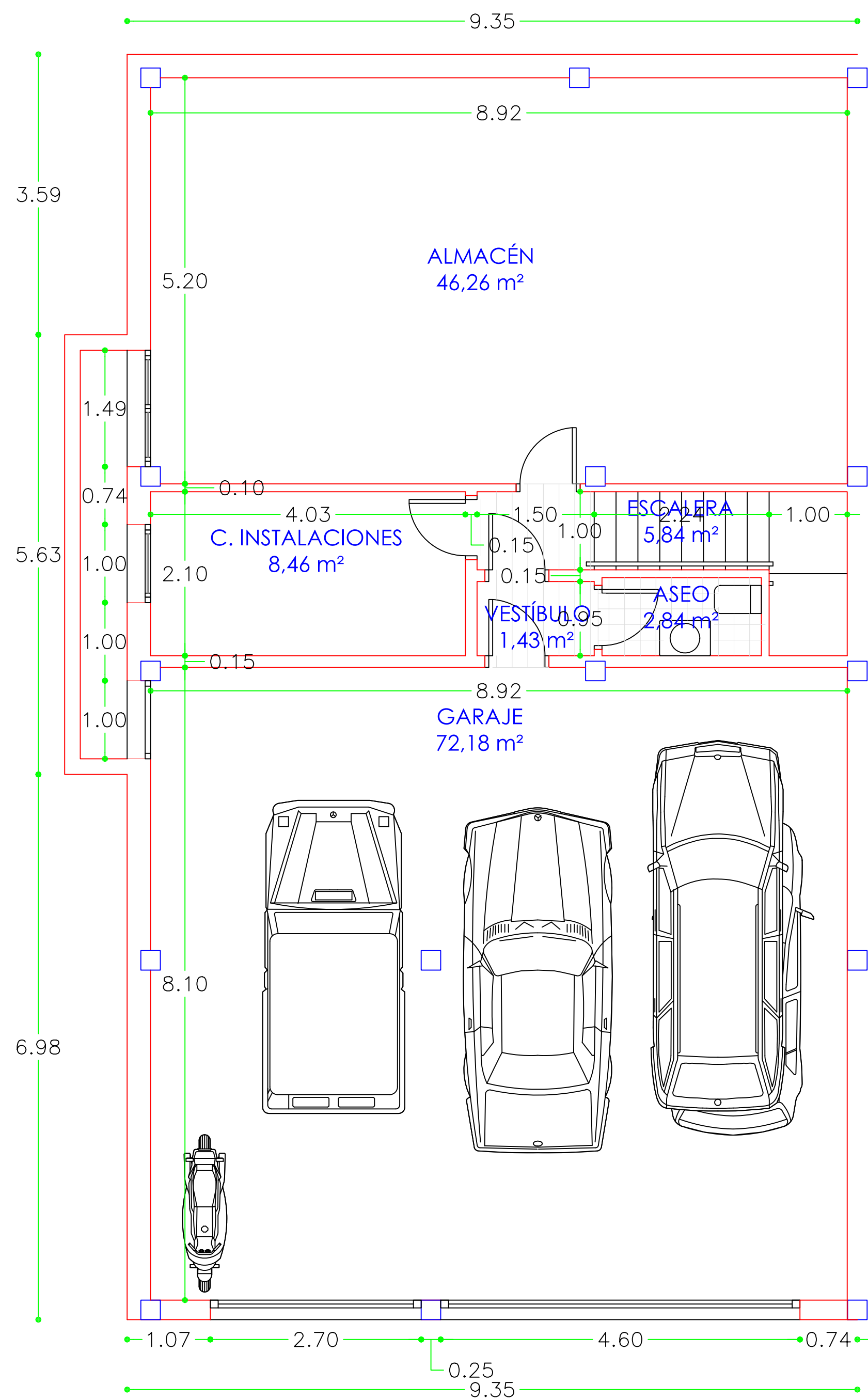
PLANTA SÓTANO
