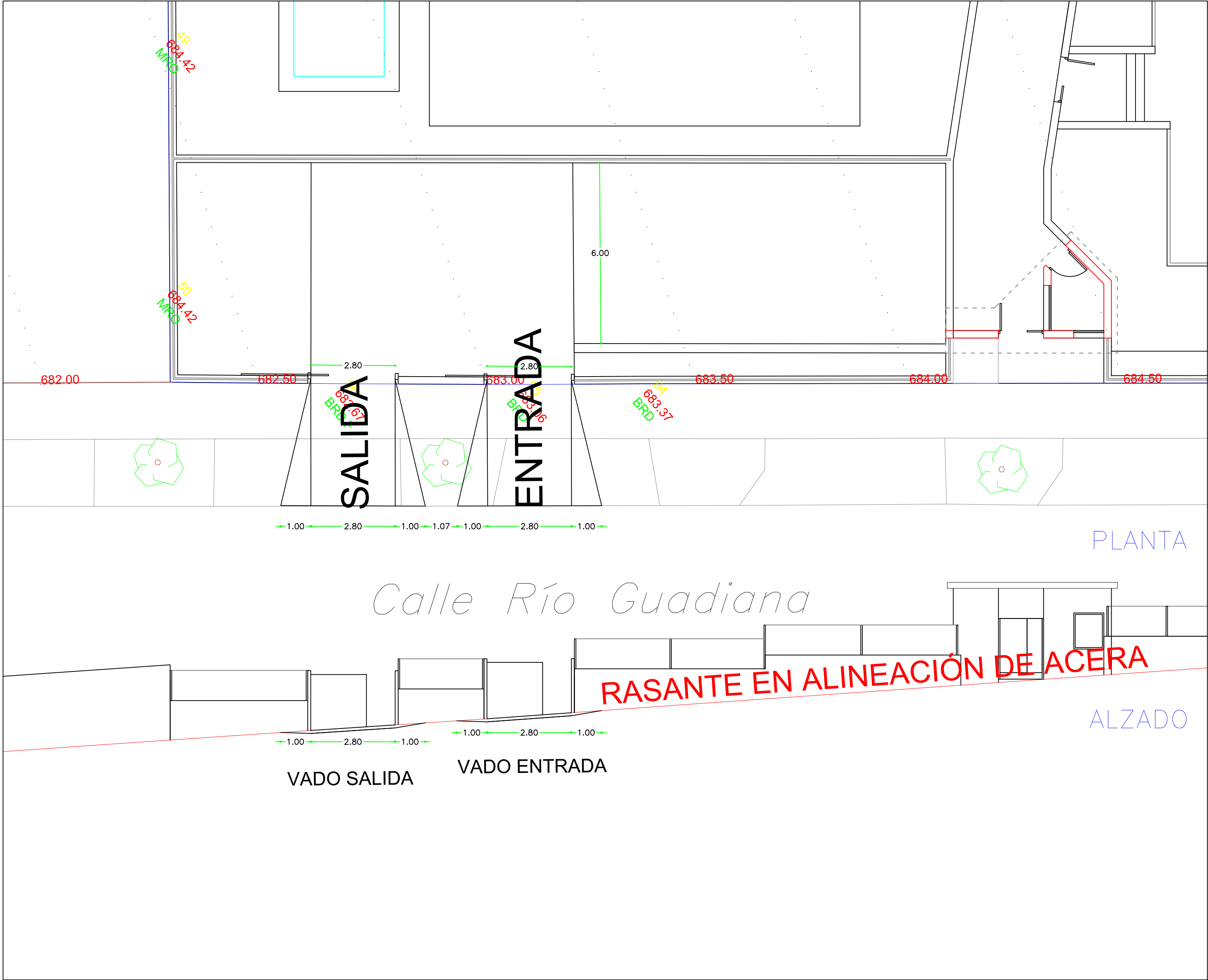
VADO GARAJE 2
