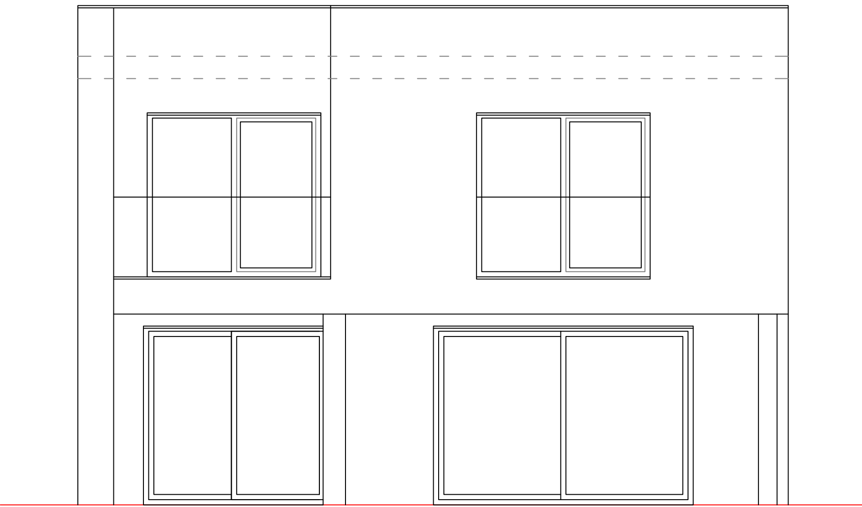
ALZADO POSTERIOR
