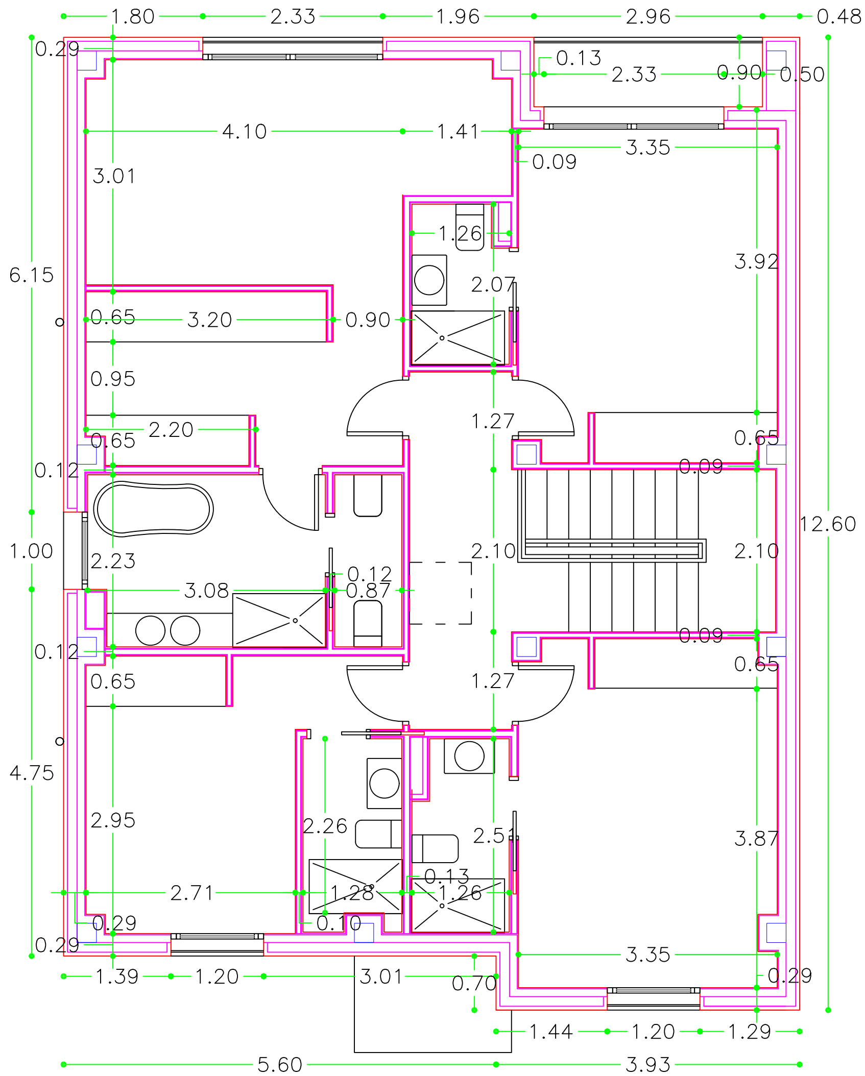
COTAS
