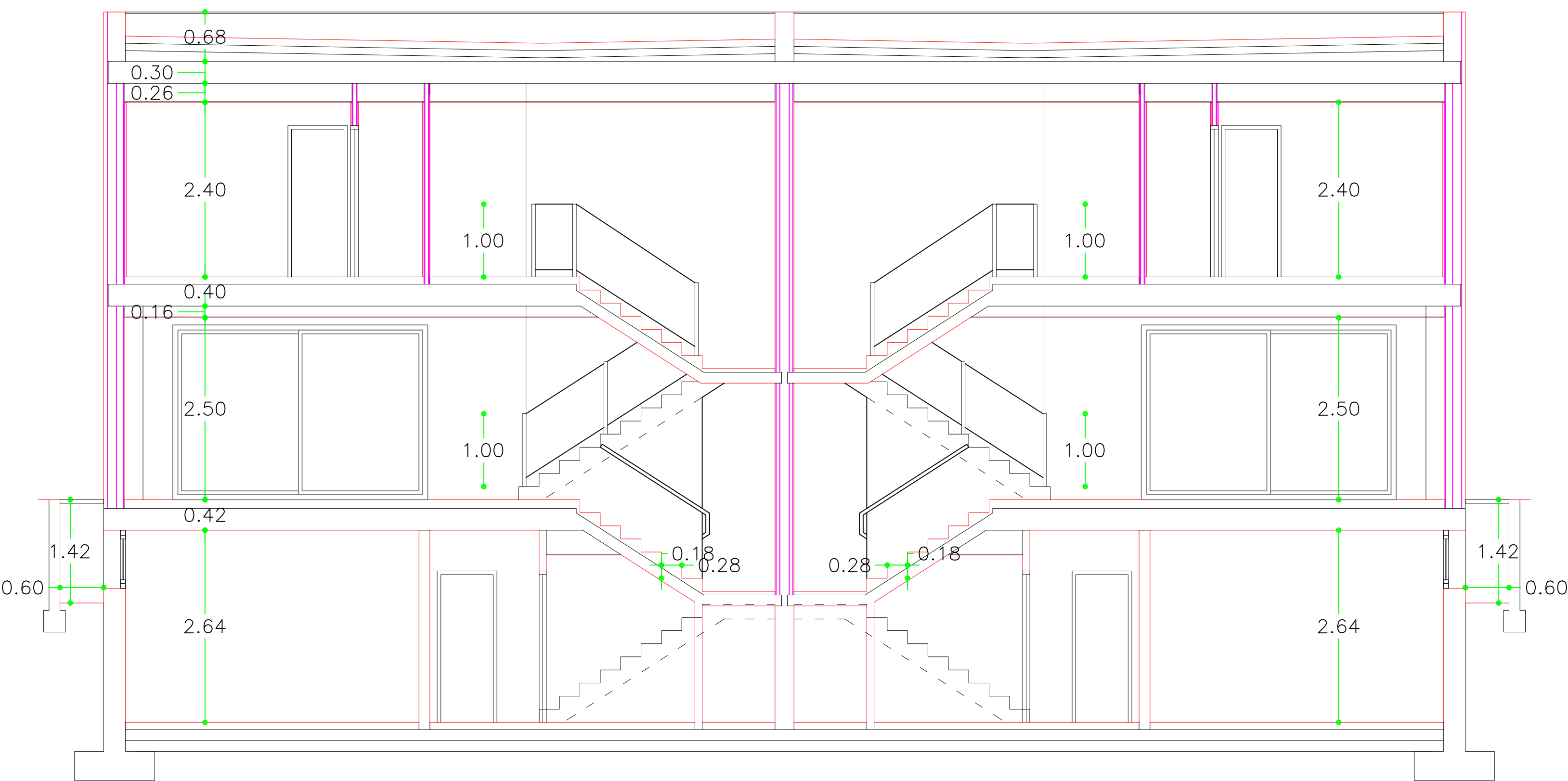
SECCIÓN TRANSVERSAL
