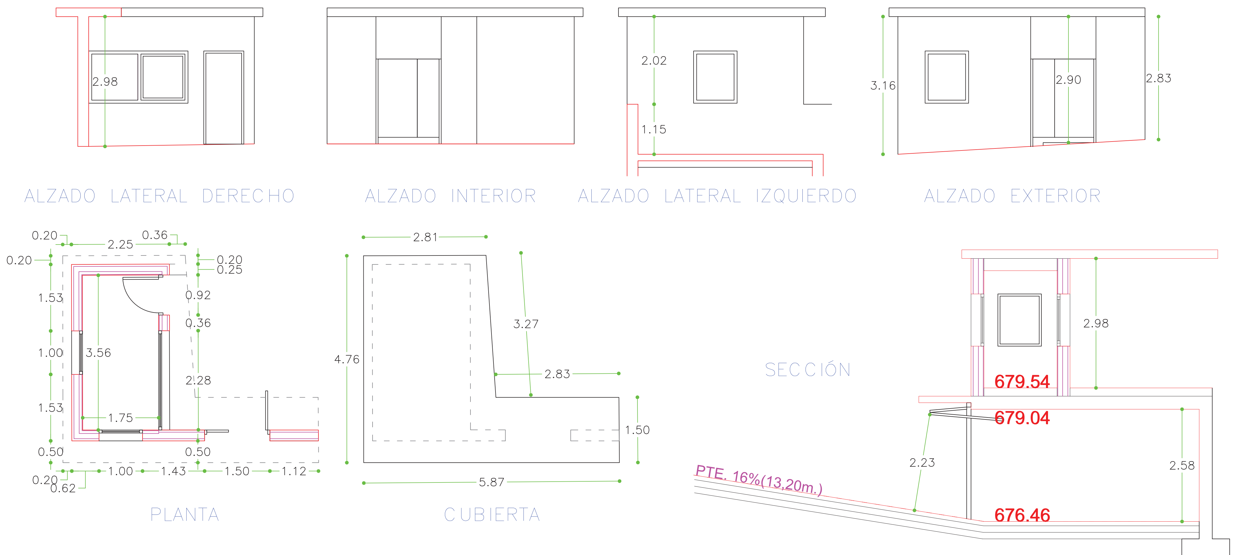
CONSERJERÍA 1
