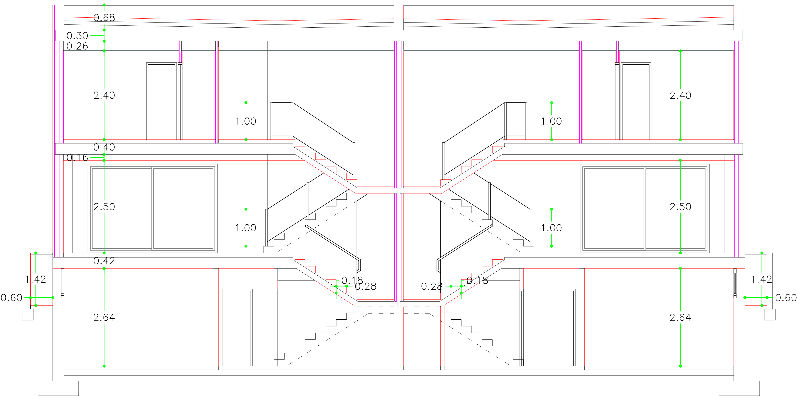
SECCIÓN TRANSVERSAL
