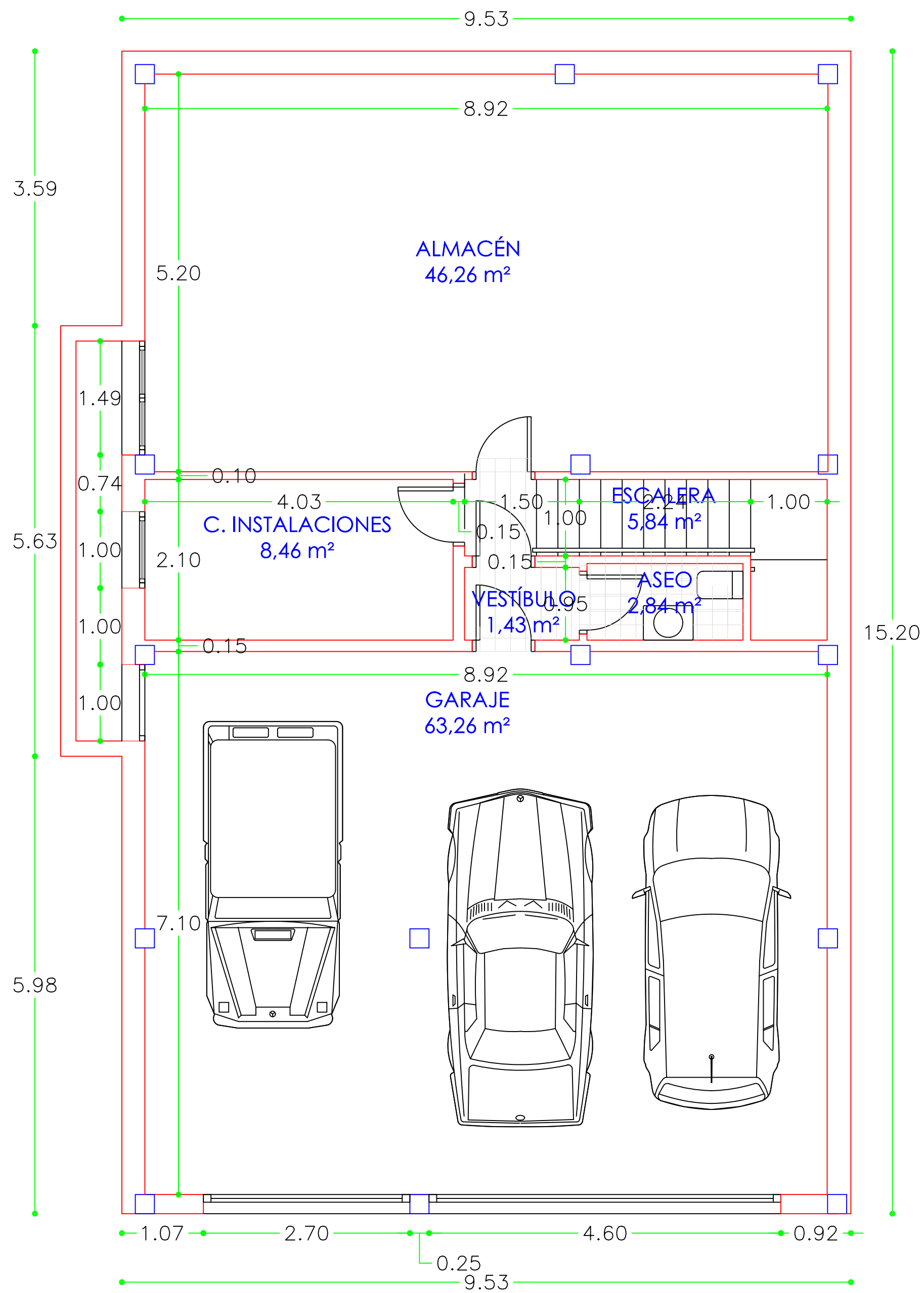
PLANTA SÓTANO
