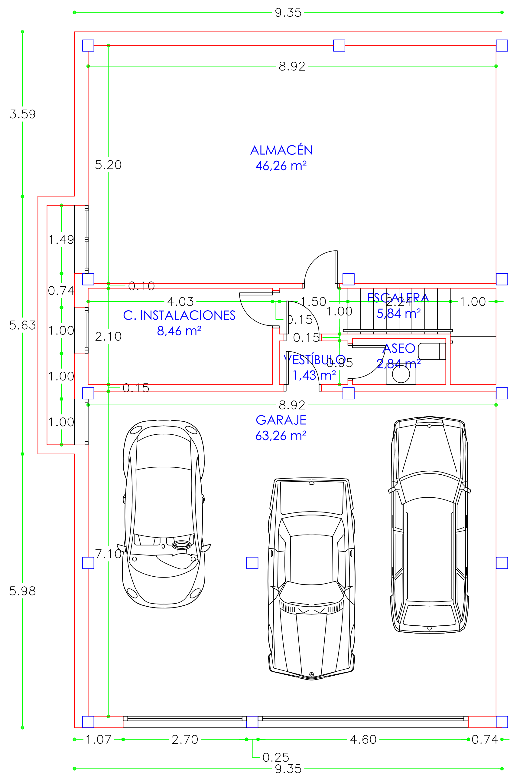
PLANTA SÓTANO
