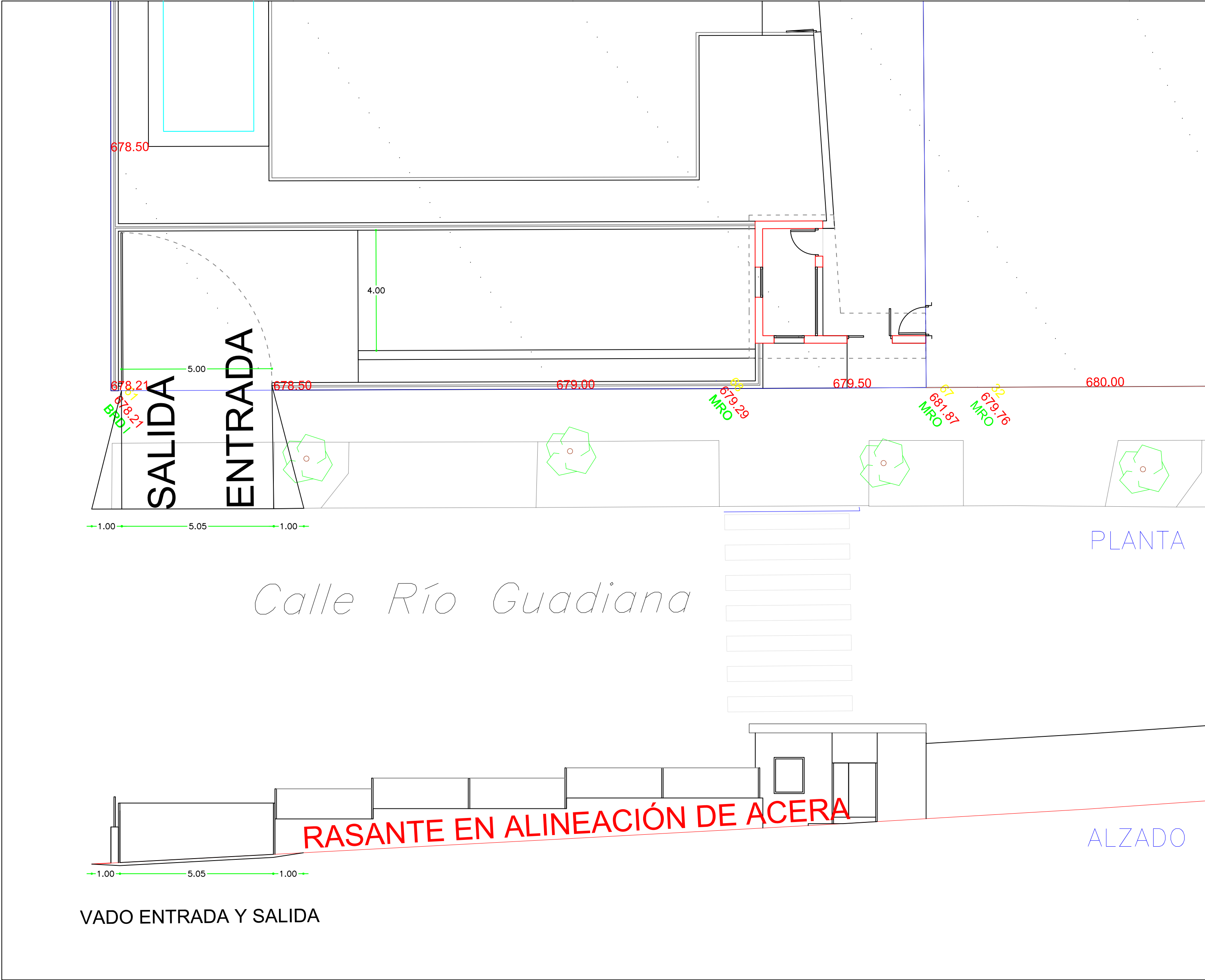
VADO GARAJE 1
