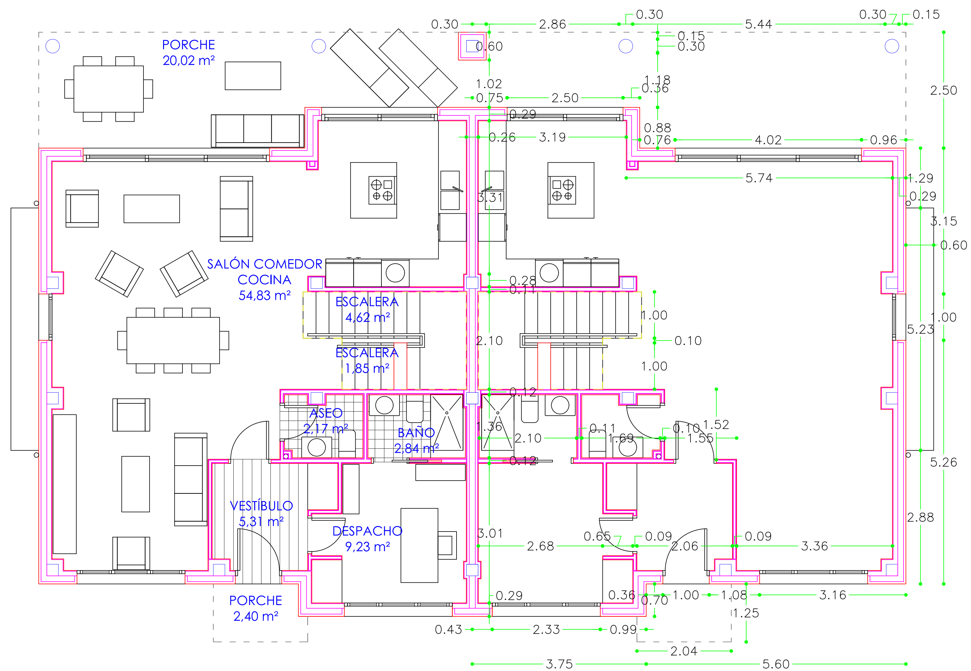
DISTRIBUCIÓN
