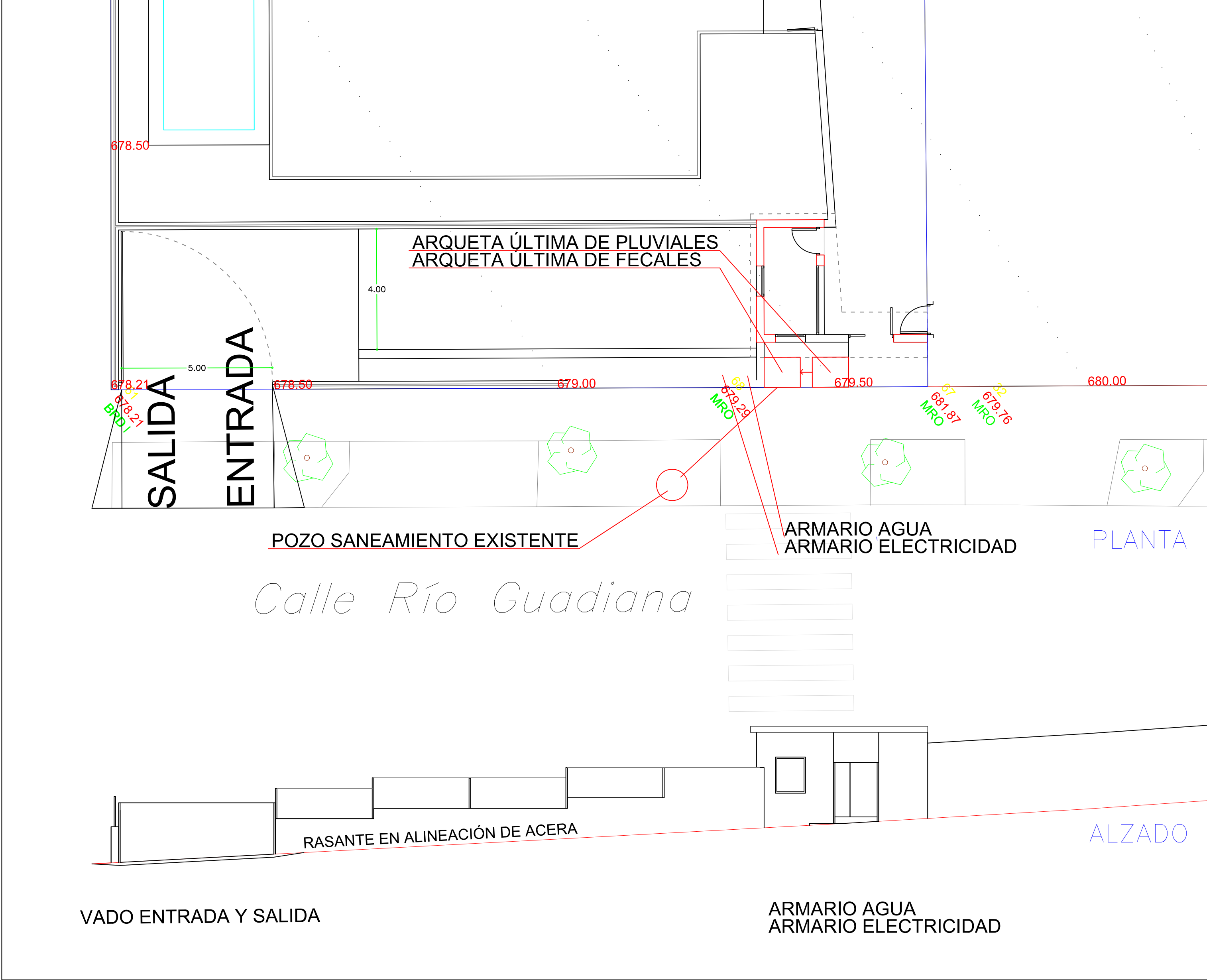
ACOMETIDAS PORTAL 1
