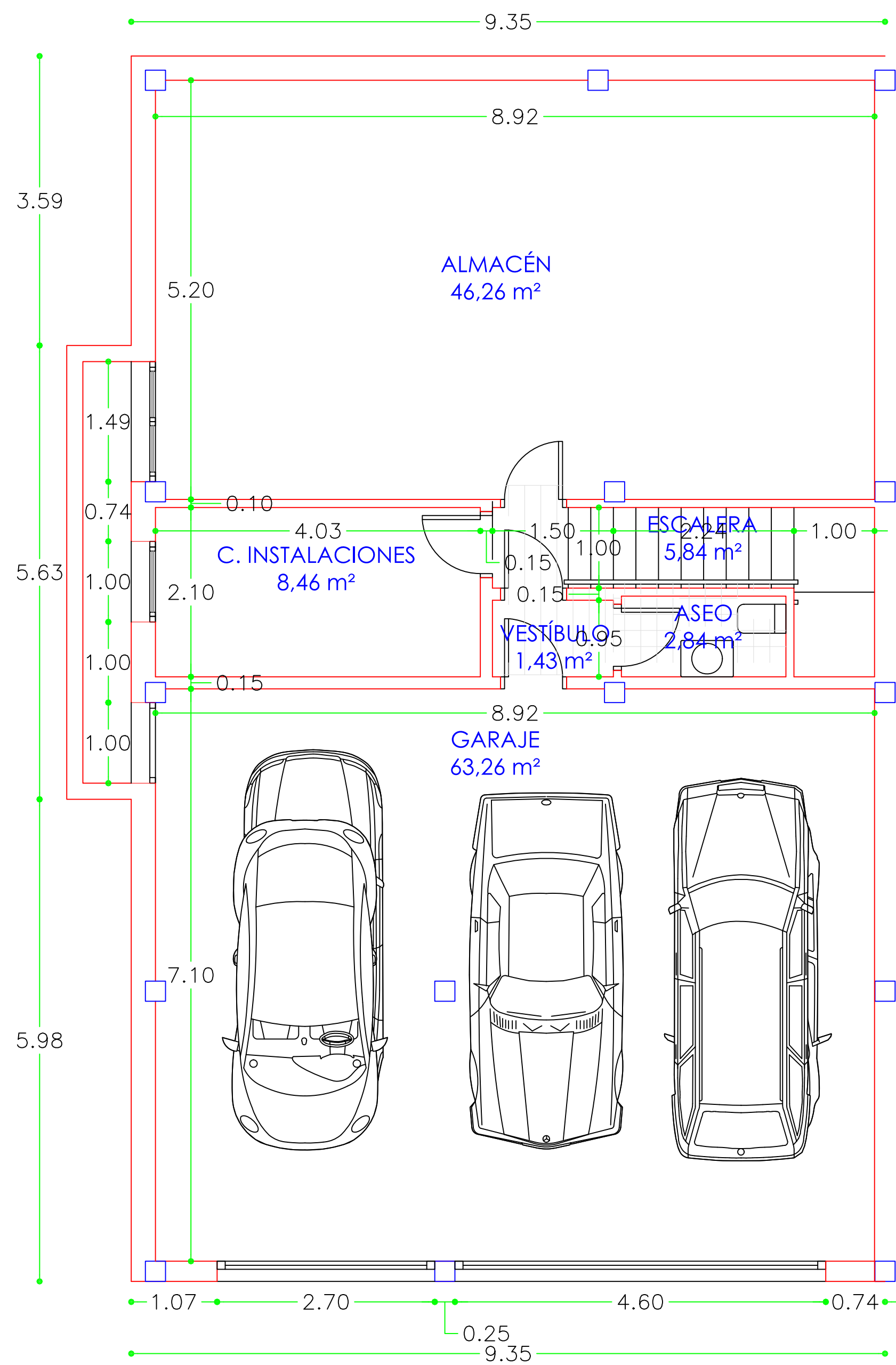
PLANTA SÓTANO
