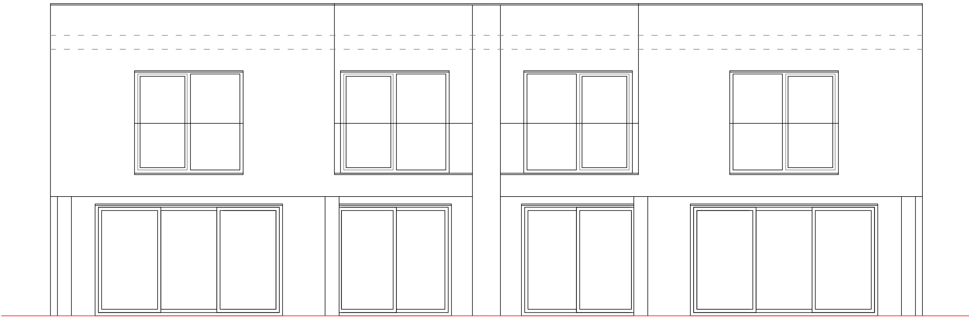
ALZADO POSTERIOR
