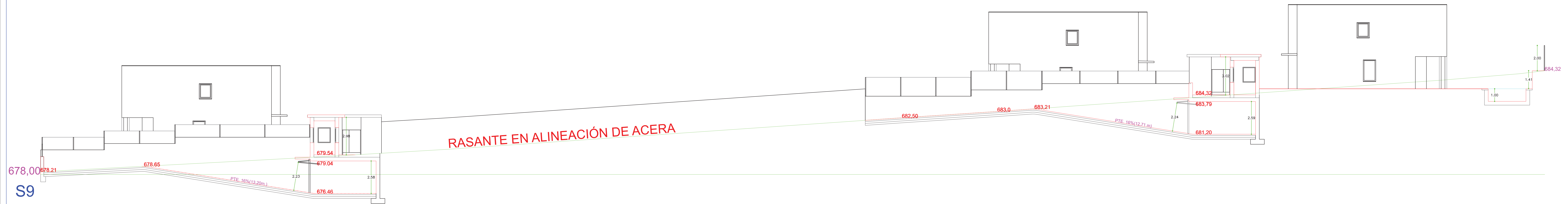
SECCIÓN POR RAMPAS
