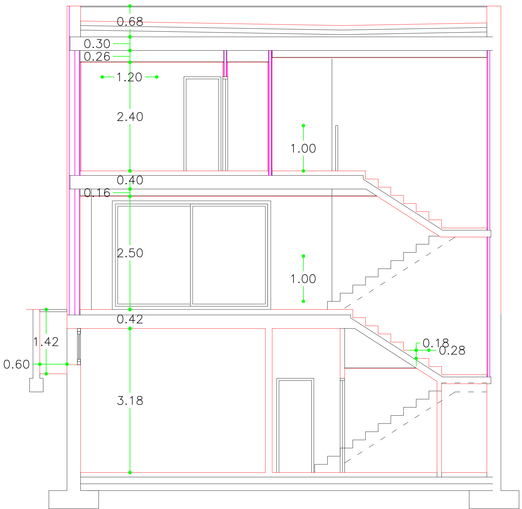
SECCIÓN TRANSVERSAL
