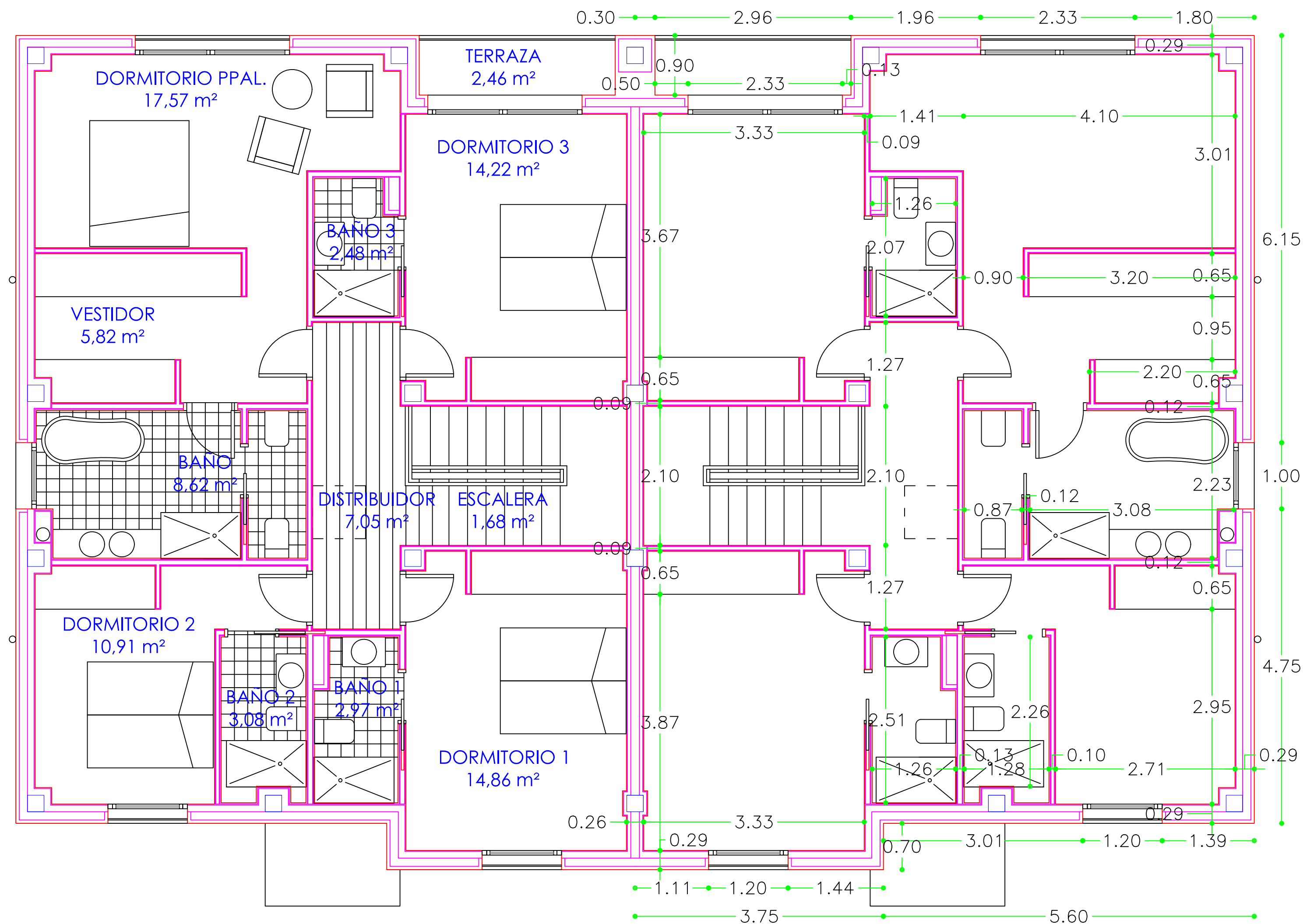
DISTRIBUCIÓN
