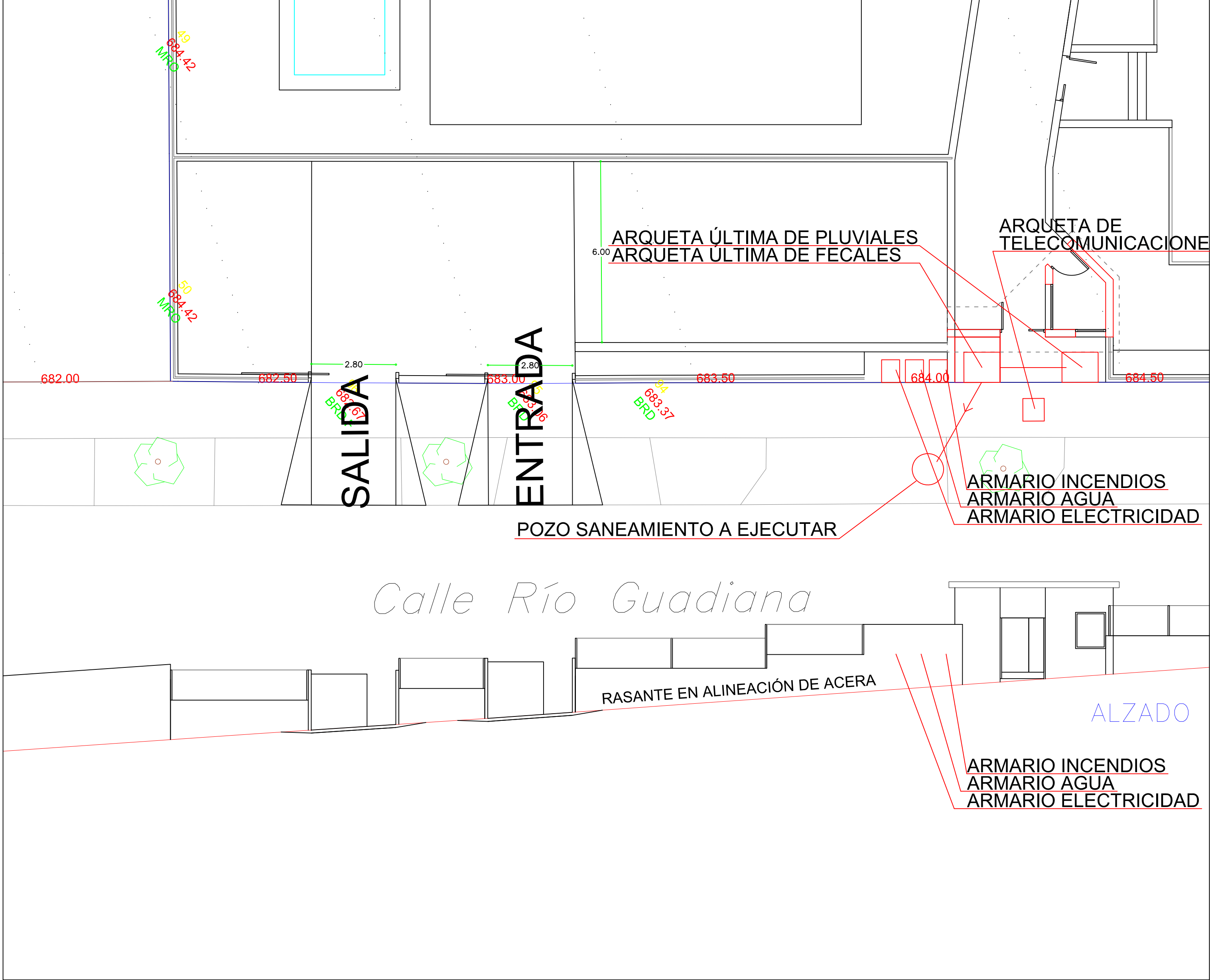
ACOMETIDAS PORTAL 2
