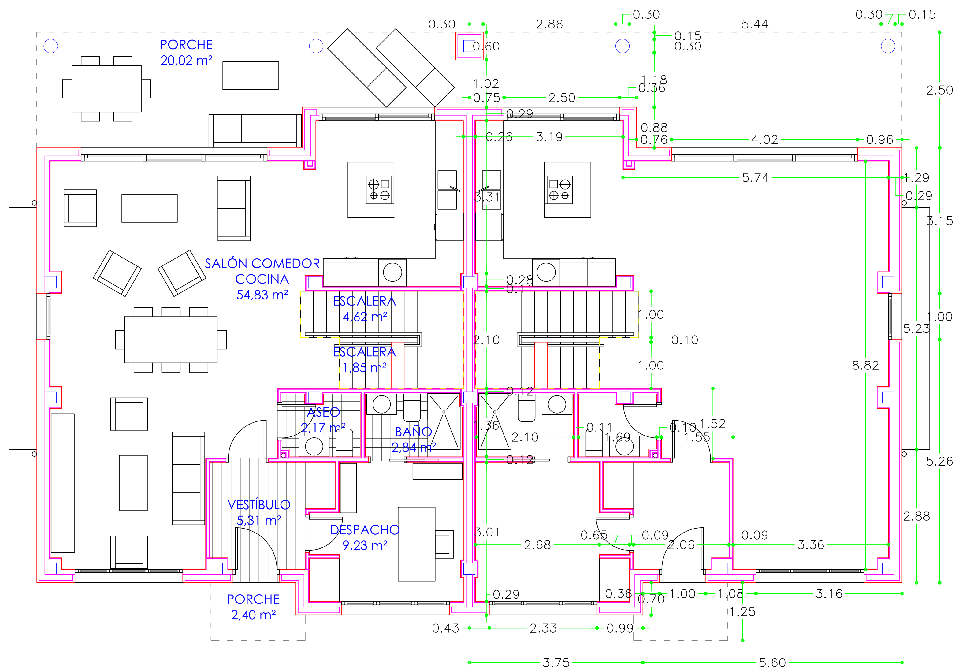
DISTRIBUCIÓN
