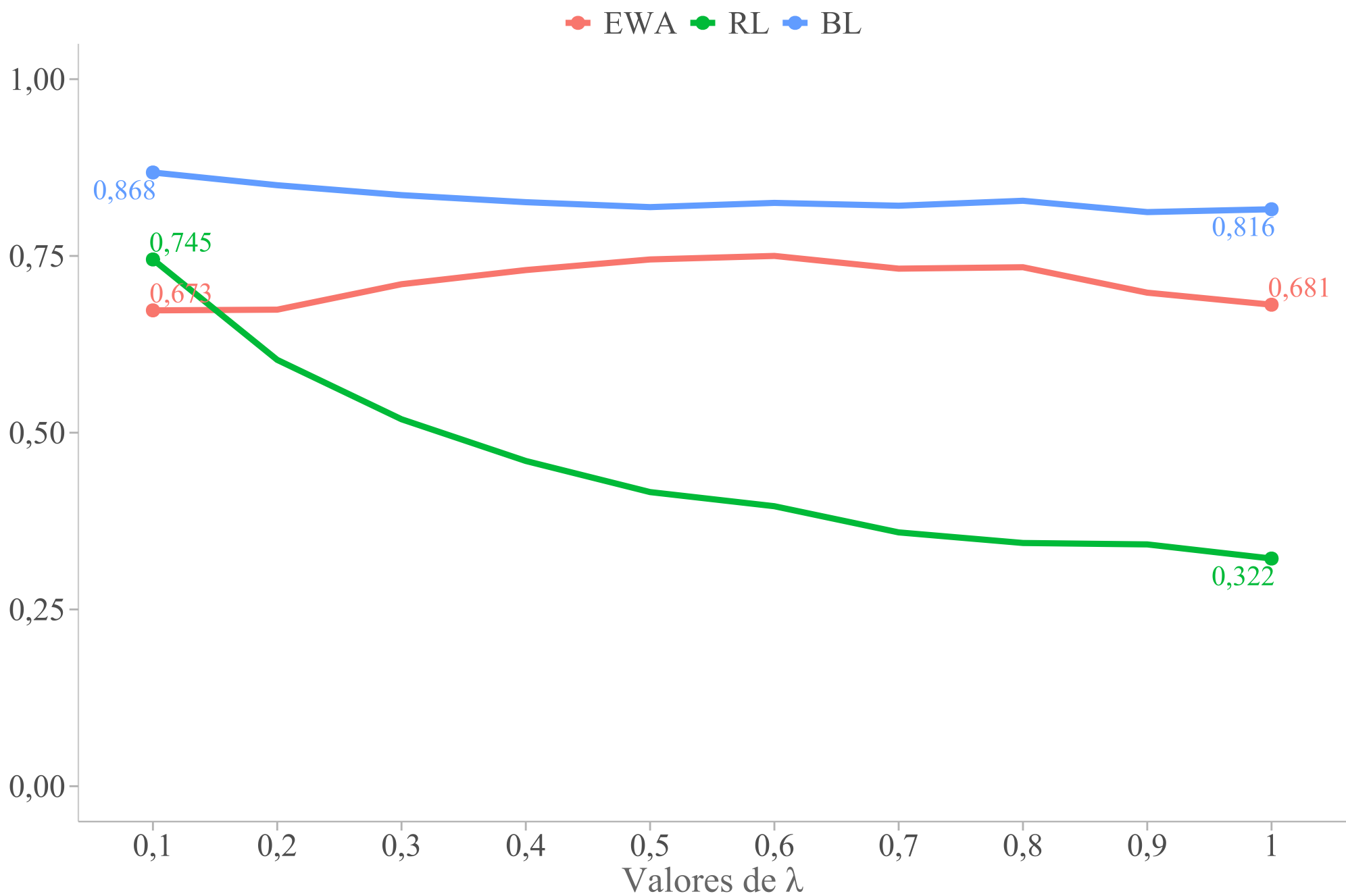
(b) MEG
