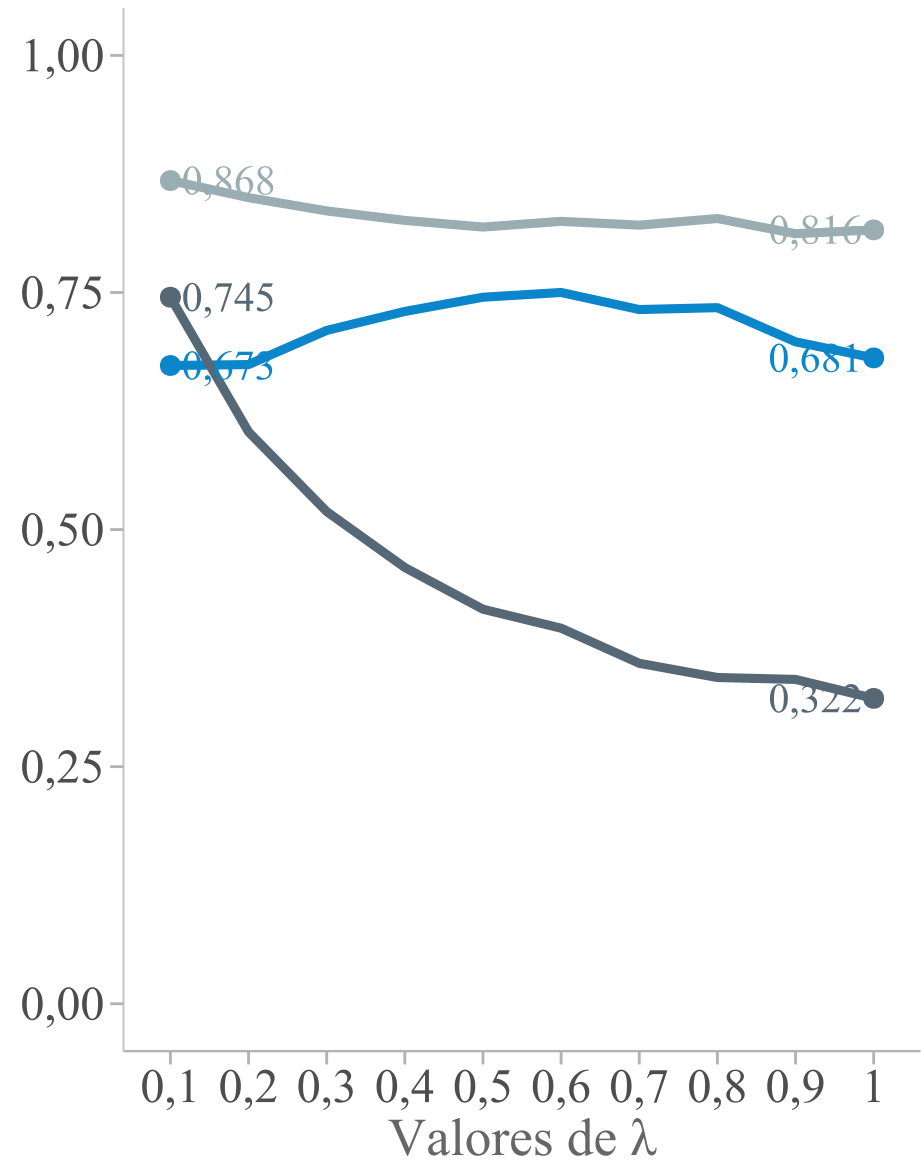
(b) MEG
