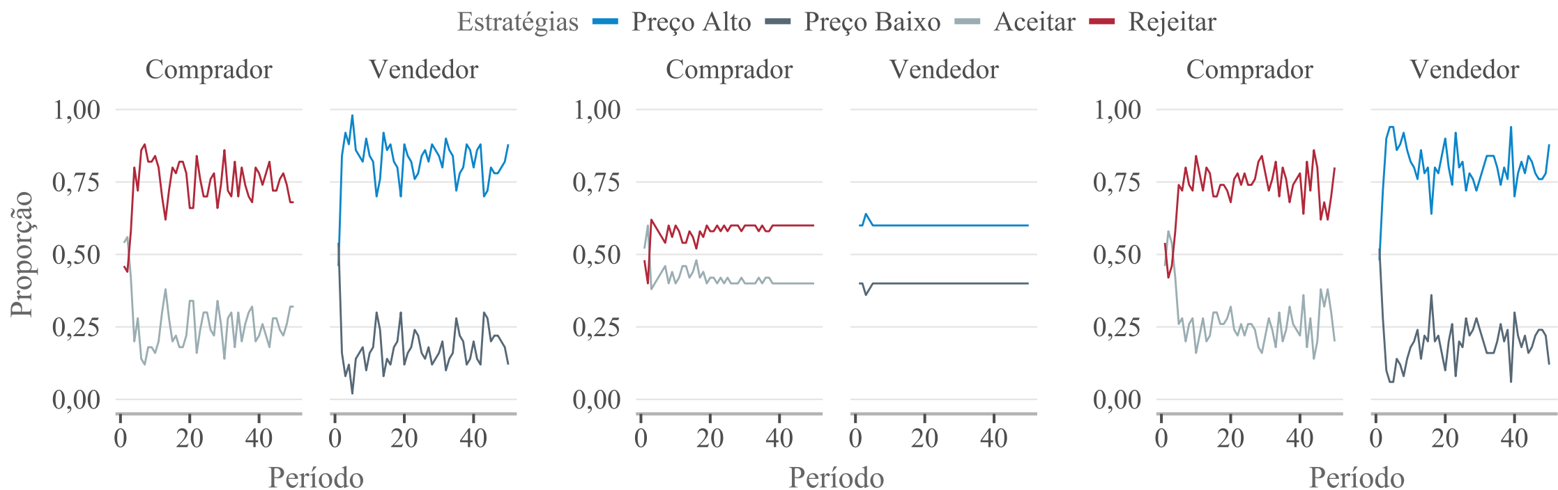
(a) EWA – BSG ( \lambda = 0,5 )
