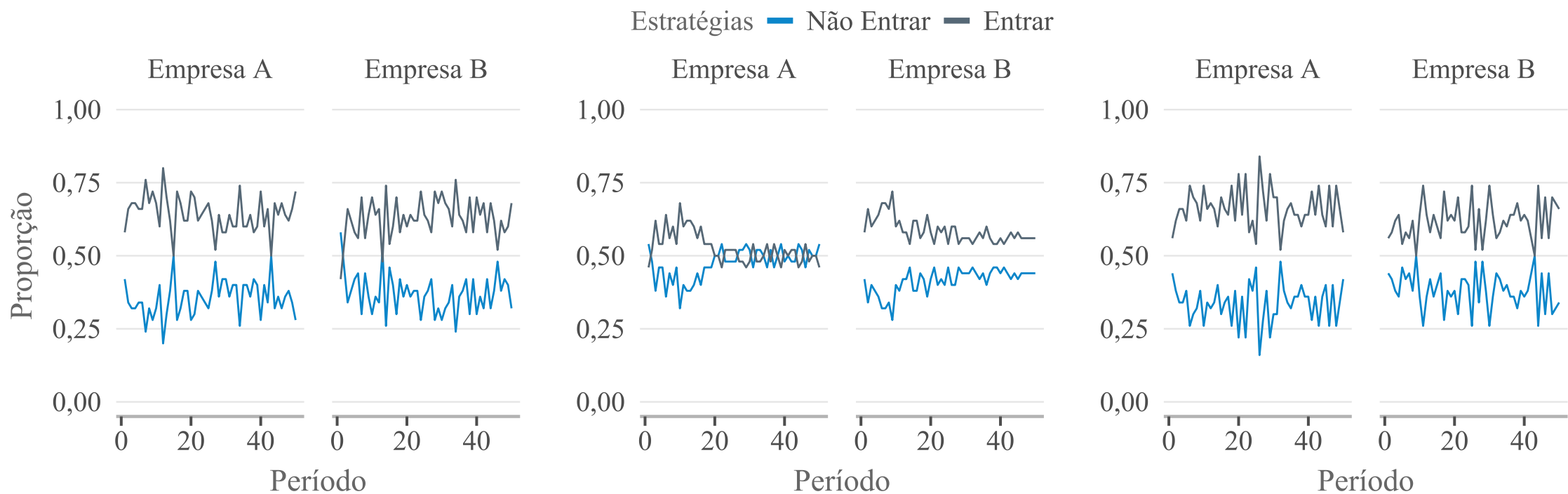
(d) EWA – MEG ( \lambda = 0,5 )
