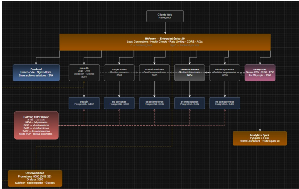
Figura 1. Diagrama de Infraestructura del Sistema
