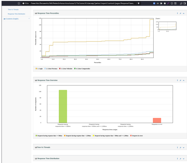
Figura 8. Distribución de percentiles de tiempo de respuesta
