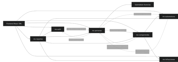
Figura 4. Relación y Comunicación entre Microservicios
