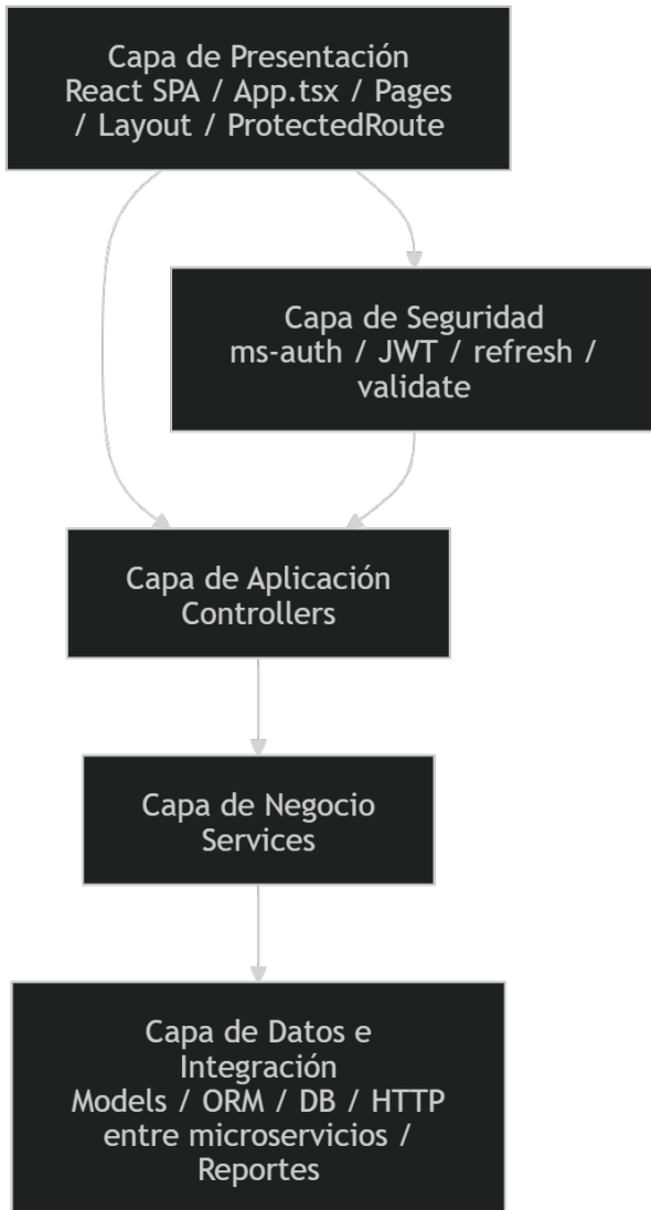
Figura 2. Diagrama de Arquitectura por Capas
