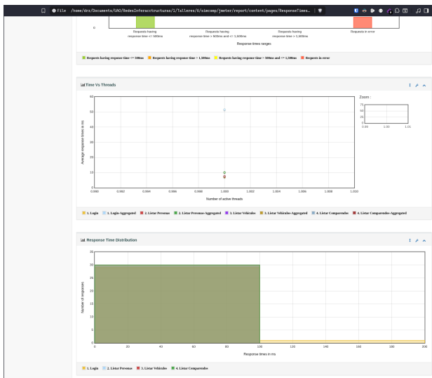
Figura 9. Frecuencia de respuesta y distribución de latencia
