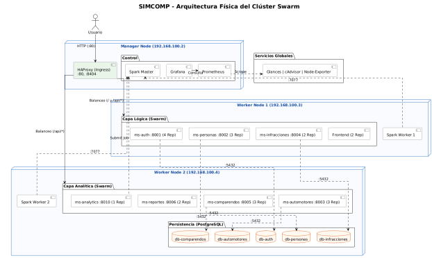
Figura 3. Diagrama de Despliegue en el Clúster Swarm
