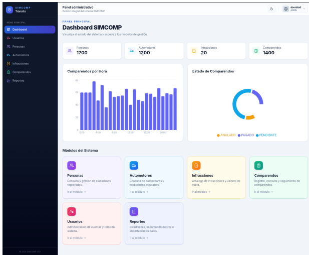
Figura 5. Interfaz de Usuario (Frontend React)
