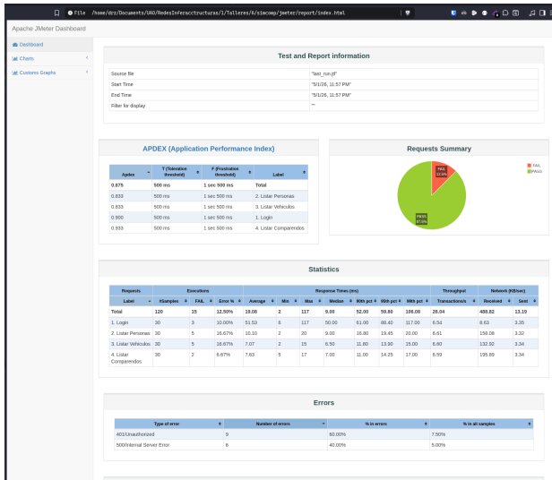
Figura 6. Métricas de rendimiento generales generadas por JMeter
