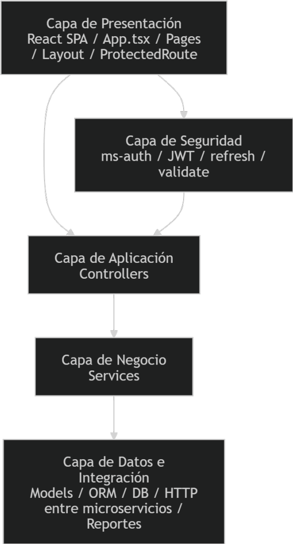
Figura 1. Diagrama de Arquitectura por Capas
