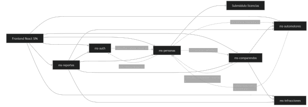
Figura 2. Relación y Comunicación entre Microservicios
