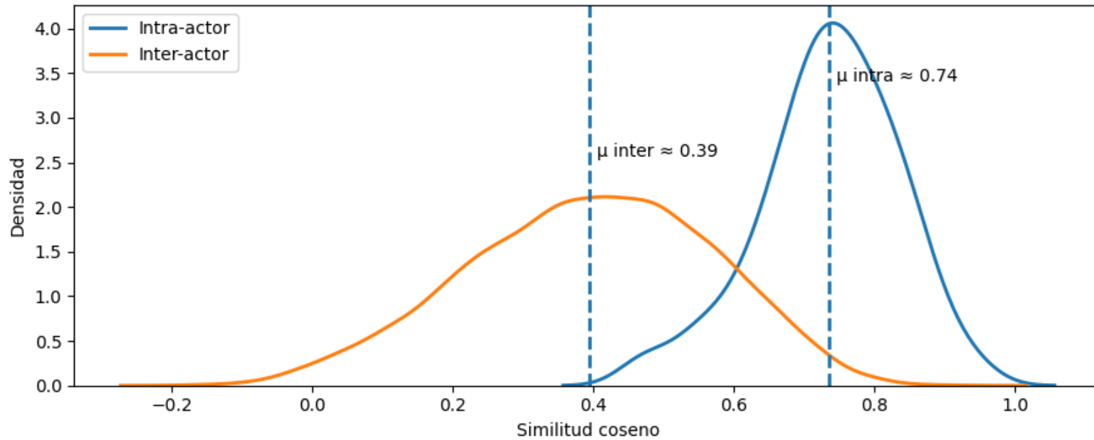
Separación de similitud coseno (densidad)
