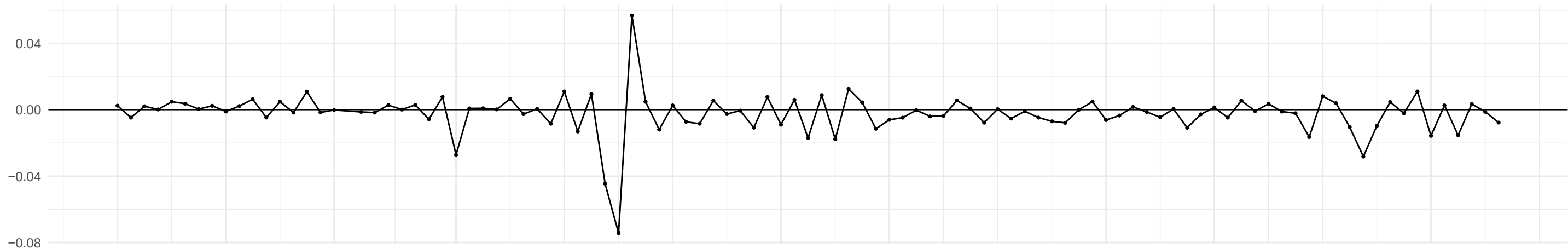
w_bar
