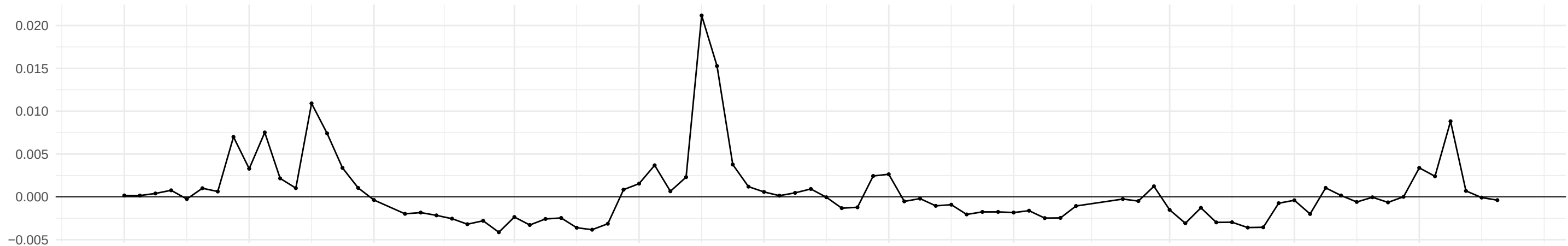
w_bar
