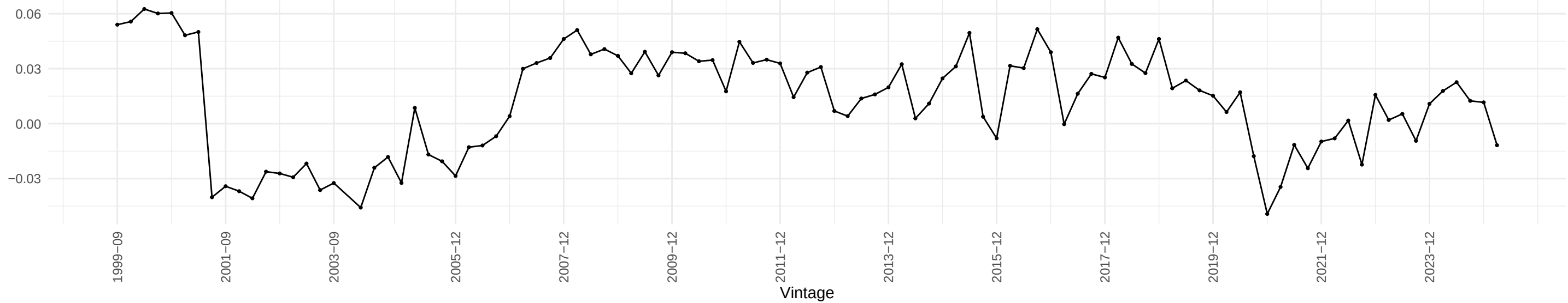
w_{\text{bar}}
